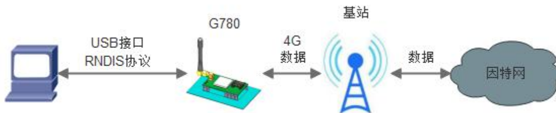
图 17 RNDIS 功能示意图
