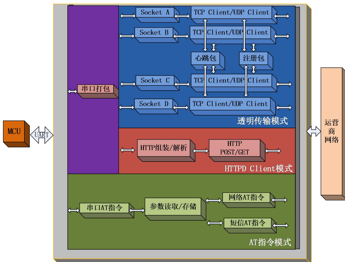
图 1 功能框图
