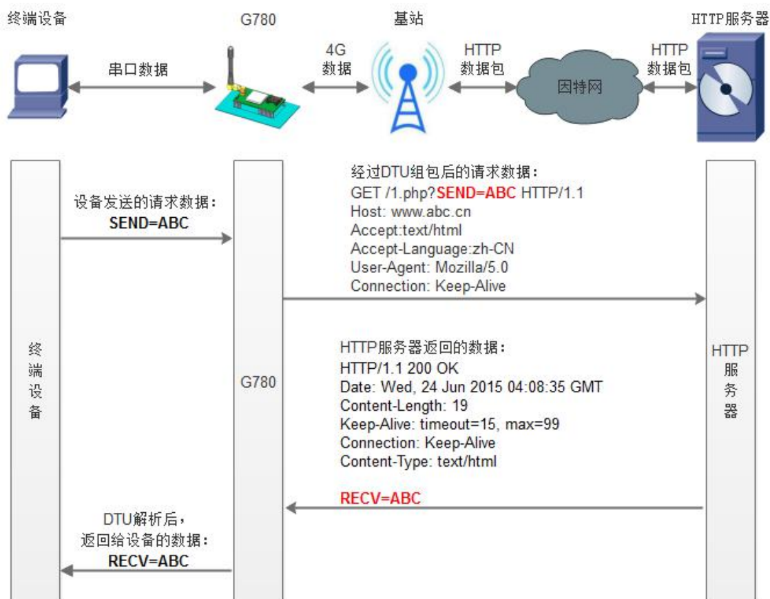
图 4 HTTPD Client 模式示意图
