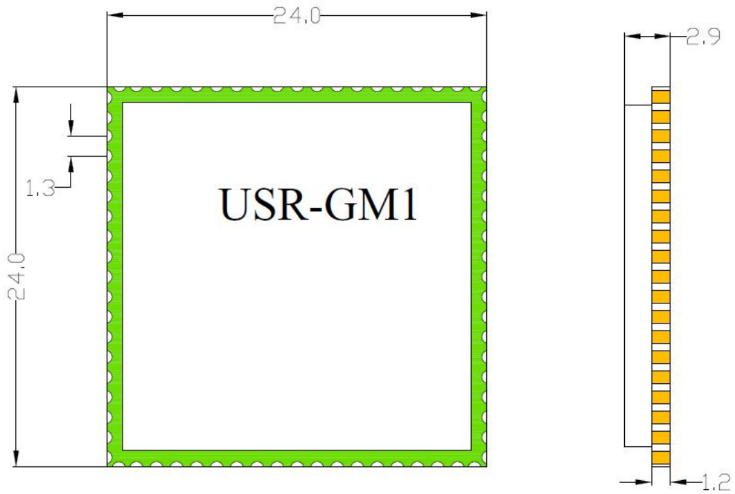
图 2 USR-GM1 尺寸图
