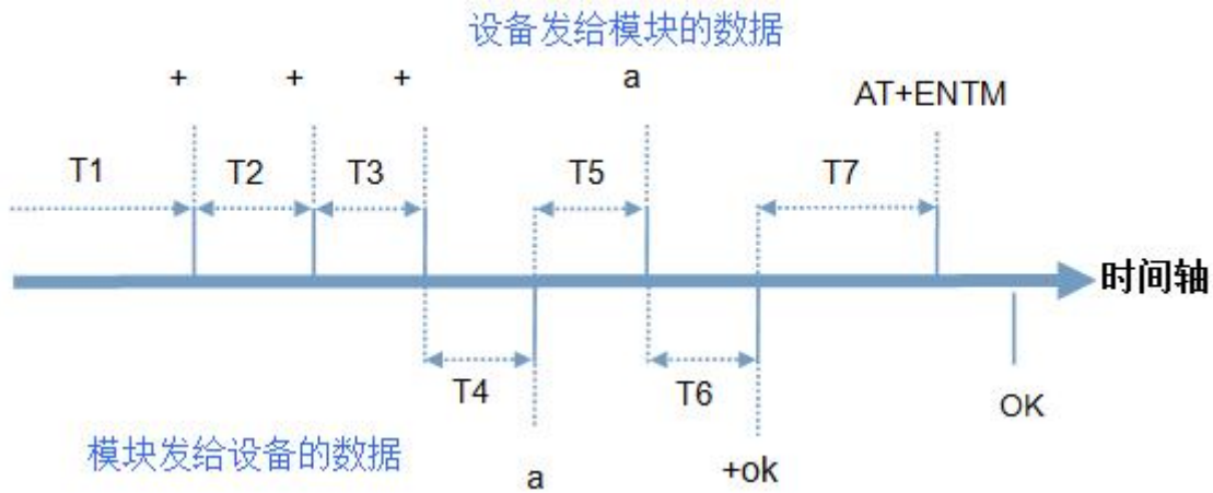
图 25 切换指令模式时序
