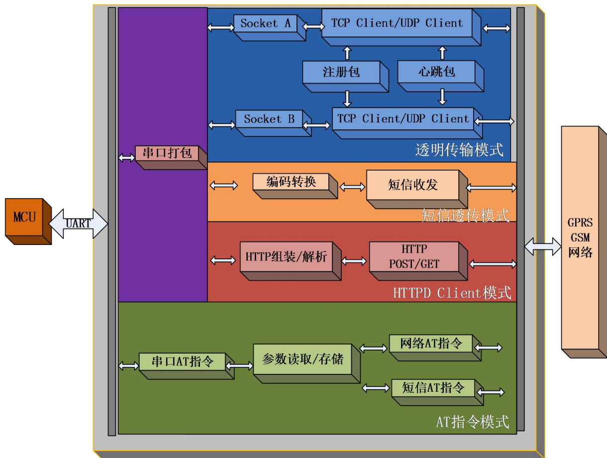
图 7 功能框图
