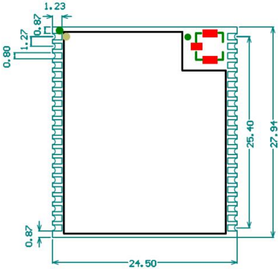
图 6 尺寸示意图
