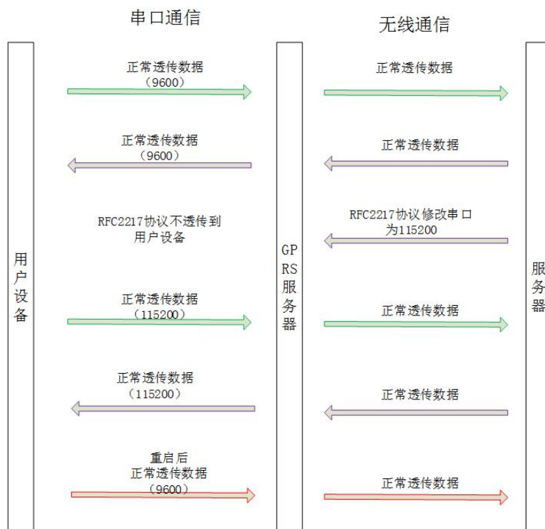
图 15 类 RFC2217 示意图
