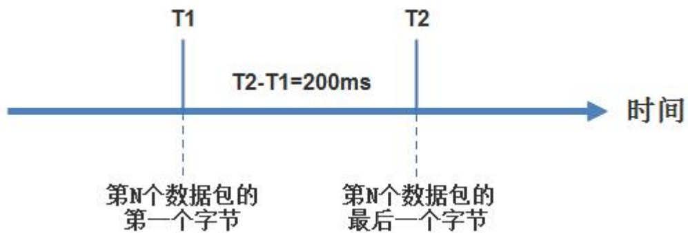
图 14 成帧机制示意图
