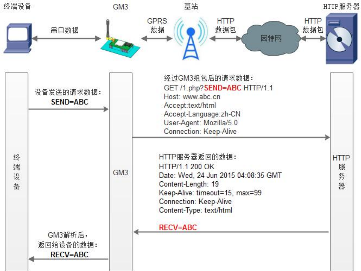
图 10 HTTPD 模式
