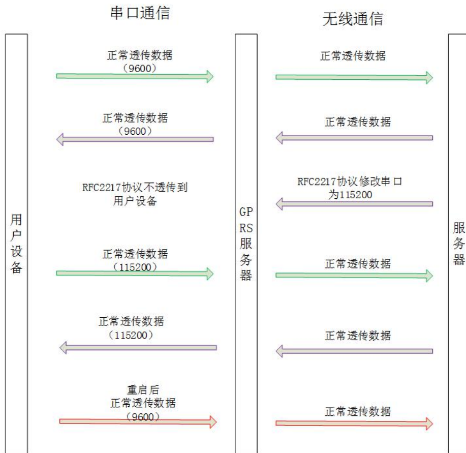
图 10 类 RFC2217 功能逻辑示意图
