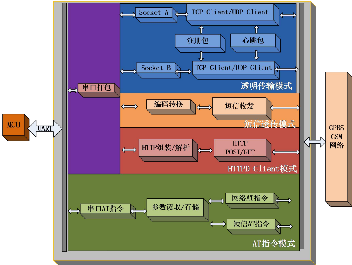
图 9 功能框图
