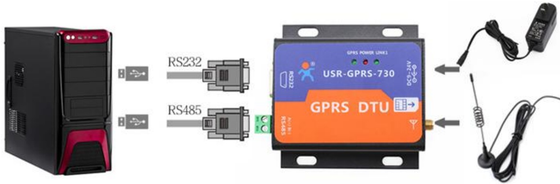
图 4 硬件连接示意图
