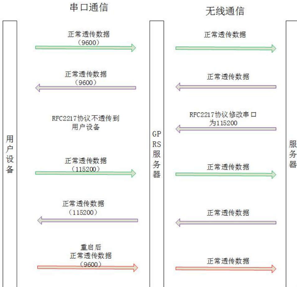
图 17 类 RFC2217 功能逻辑示意图
