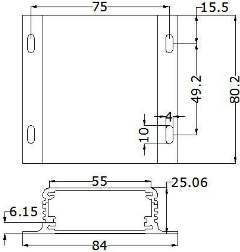
图 8 USR-GPRS232-730 尺寸图
