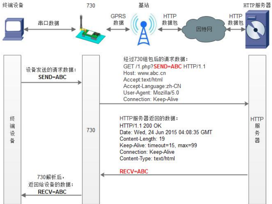
图 12 HTTPD 模式
