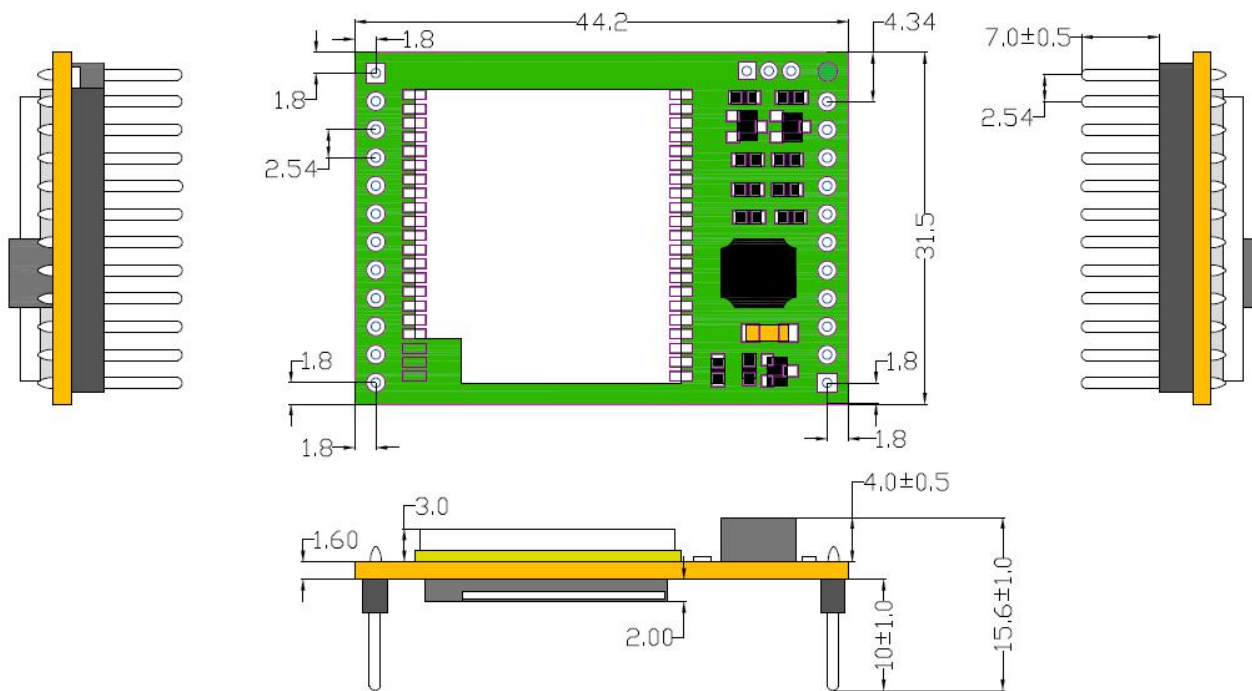
图 7 USR-GPRS232-7S3 尺寸图
