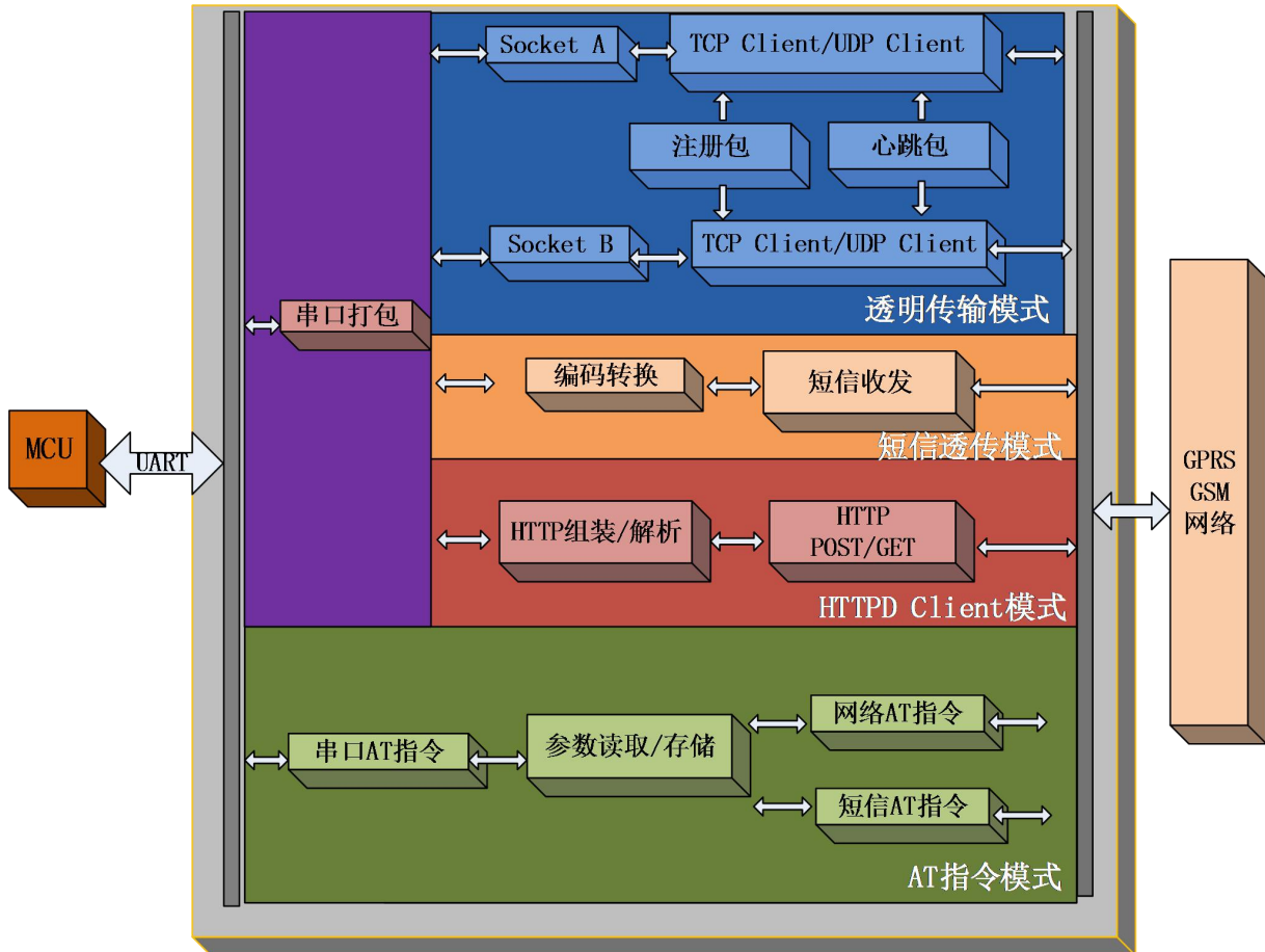
图 8 功能框图
