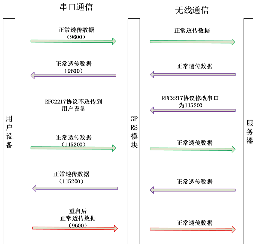
图 16 类 RFC2217 功能逻辑示意图
