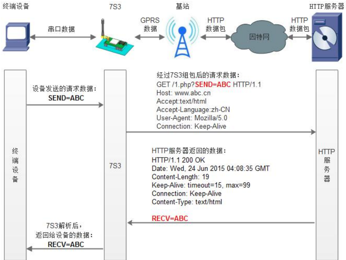
图 11 HTTPD 模式
