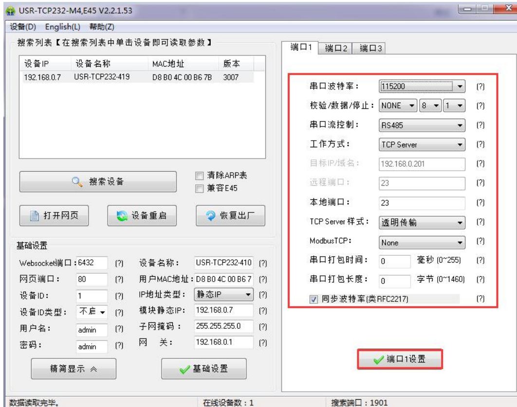
图 15 软件设置参数—端口 1 设置
