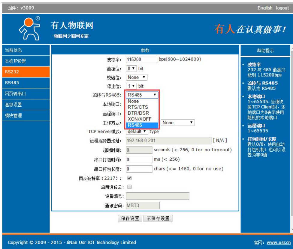
图 9 流控设置界面
