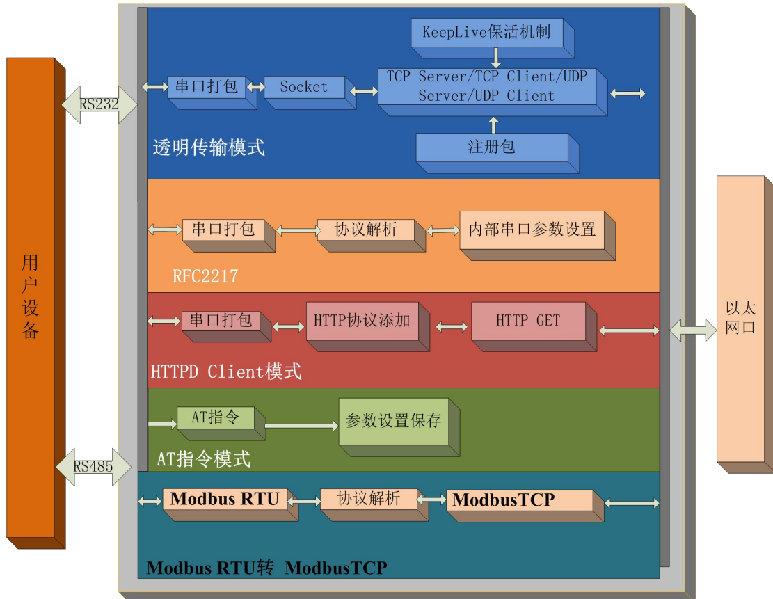
图 6 419 功能框图
