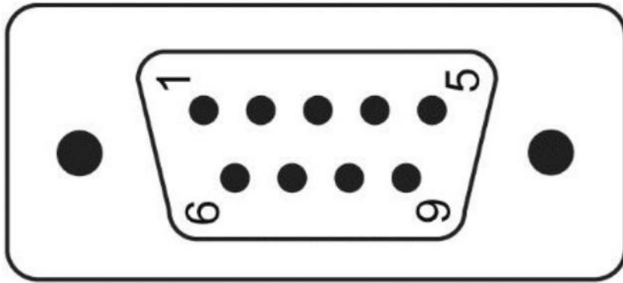
图 5 口引脚图示
