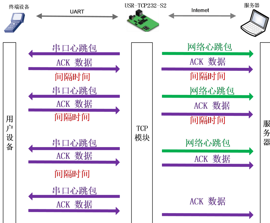
图 28. 心跳包功能示意图
