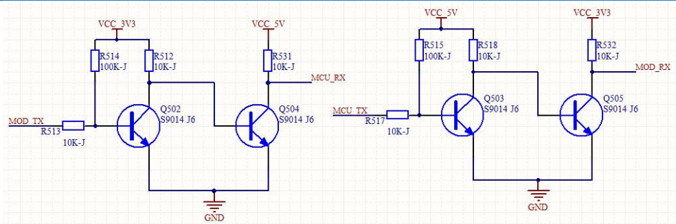
3.3V—5V 电压转换电路
