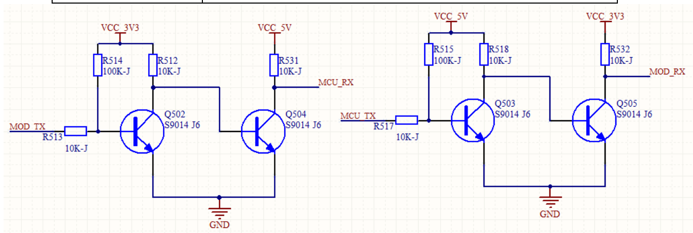
图 1-1 电压匹配电路
