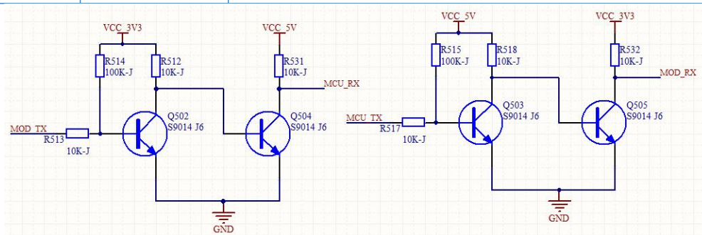
3.3V—5V 电压转换电路
