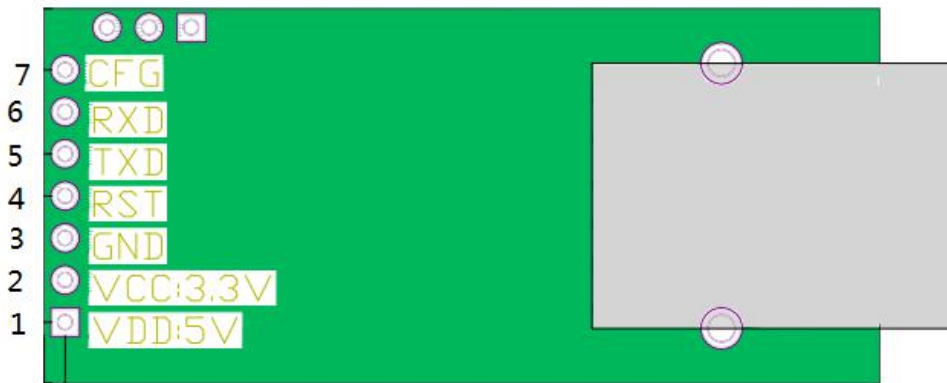
USR-TCP232-T2 接口定义
