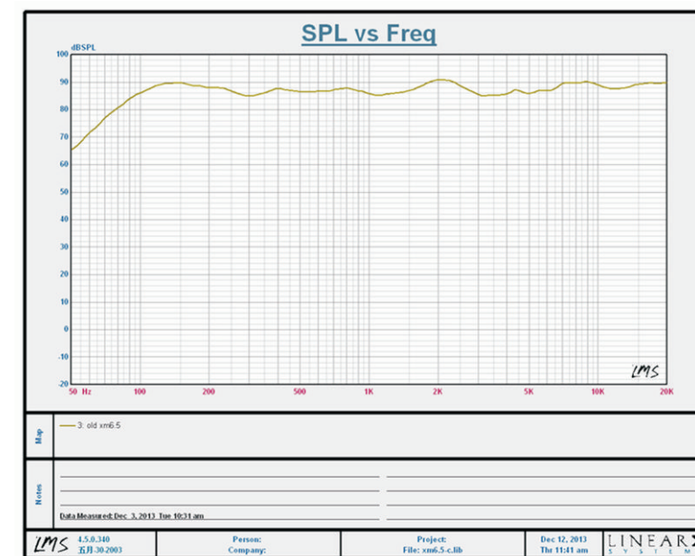
音箱频响曲线
