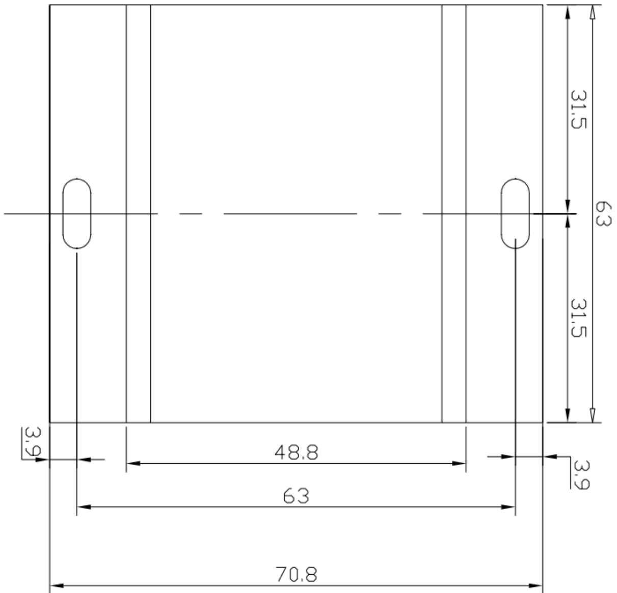
图 2 底面尺寸图(单位: mm)
