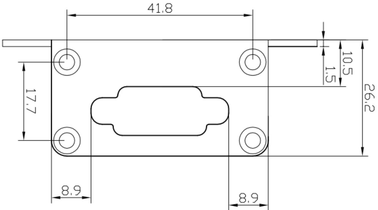
图 1 侧面尺寸图(单位: mm)
