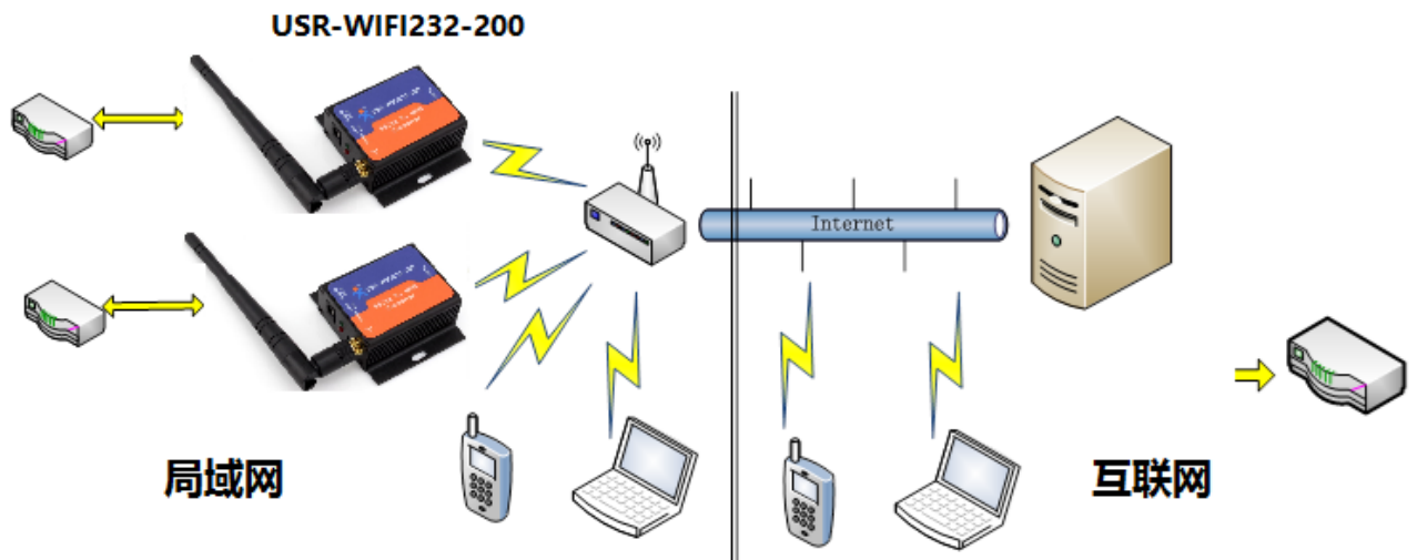
图 6 远程连接应用图示
