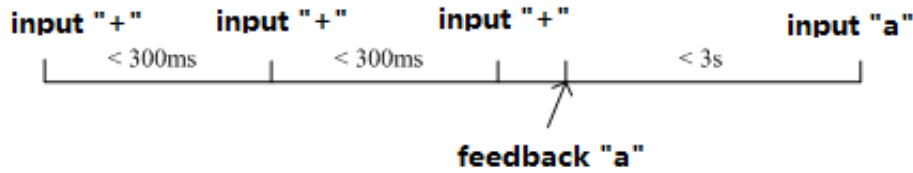
图 11 ‘+++、‘a’时序要求
