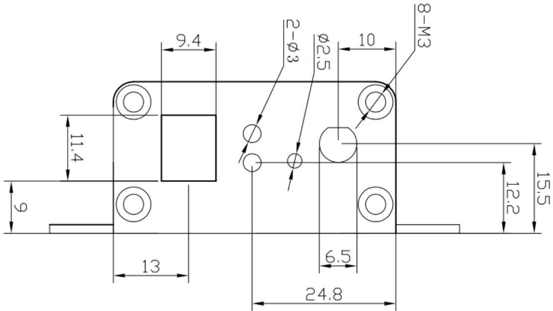
图 8 侧面尺寸图(单位: mm)
