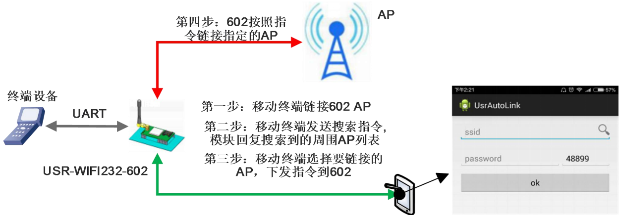
图 26 usr-link 框图
