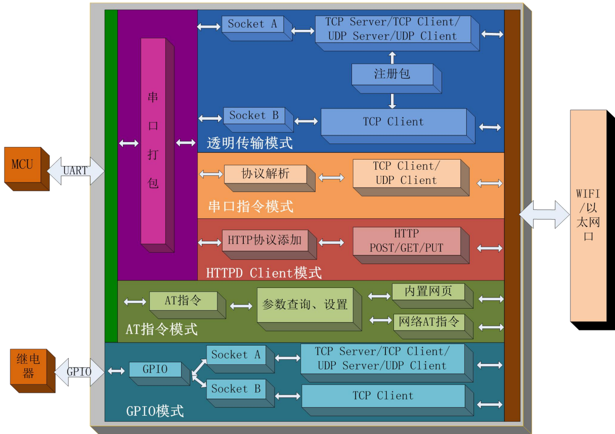
图 8 USR-WIFI232-A2 功能框图
