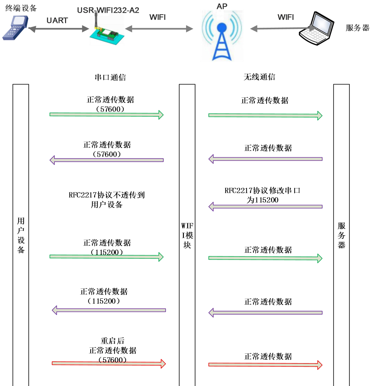
图 29 类 RFC2217 自动波特率框图
