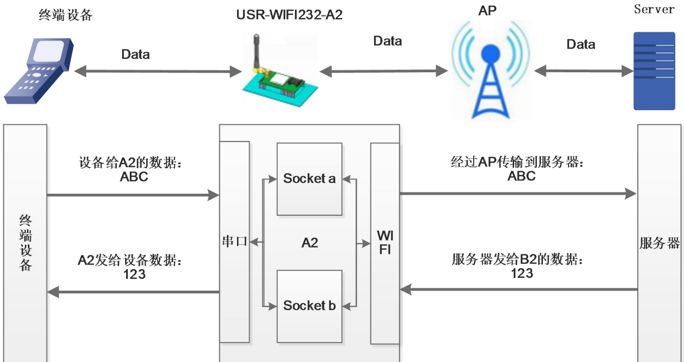
图 16 透明传输功能框图
