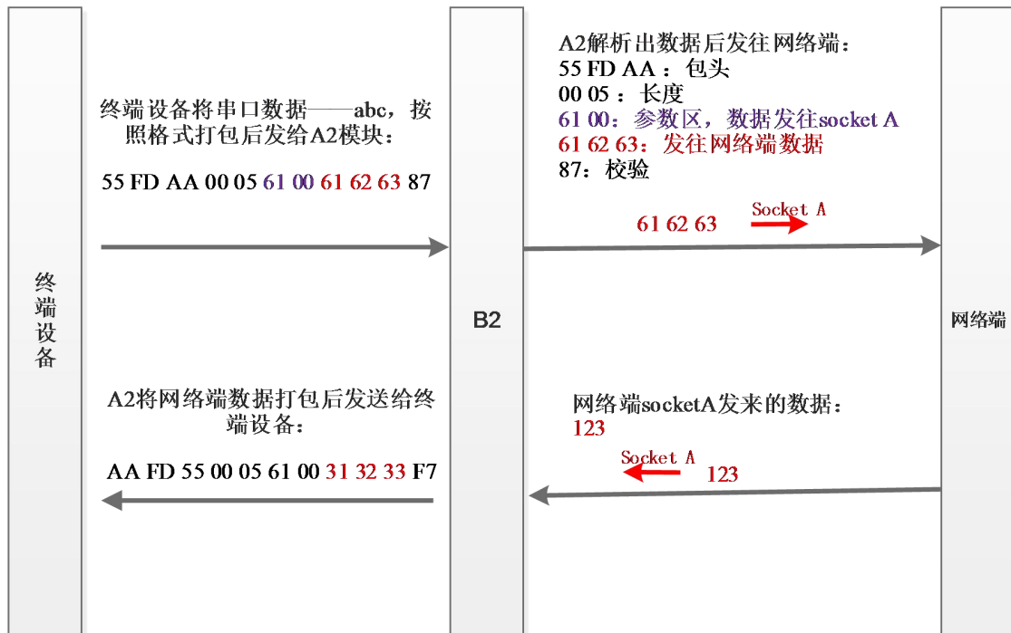
图 35 套接字分发框图
