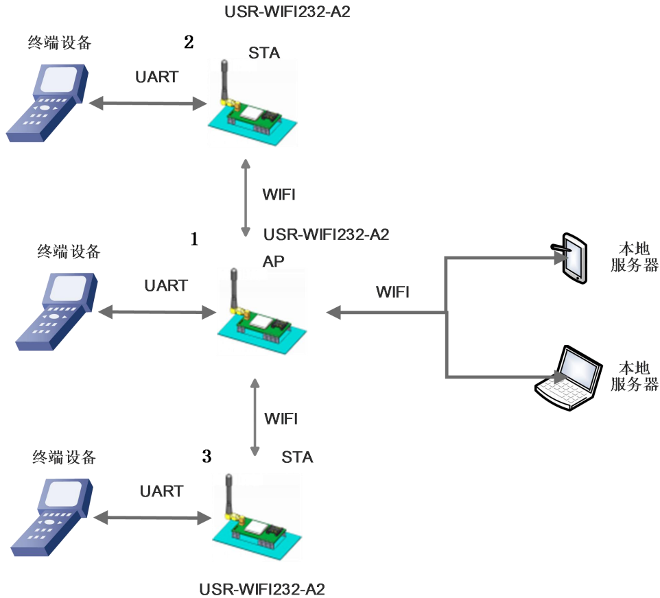
图 12 USR-WIFI232-A2 自组网 2
