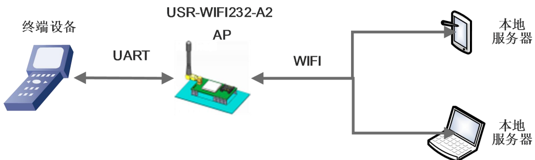
图 11 USR-WIFI232-A2 自组网 1
