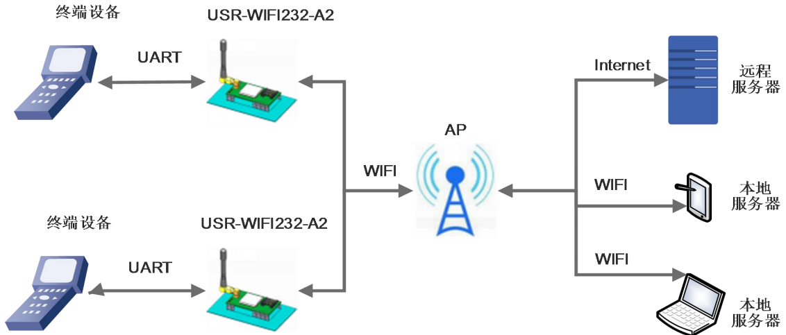
图 10 STA 方式组网
