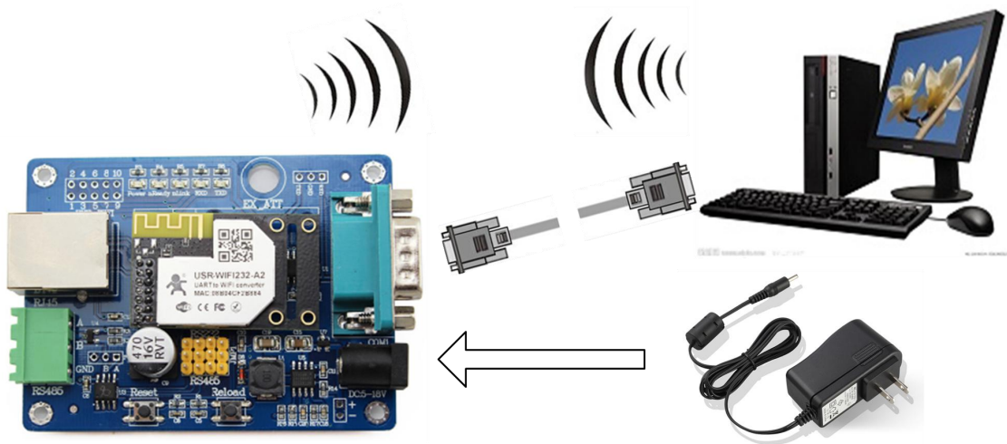
图 1 硬件连接示意图
