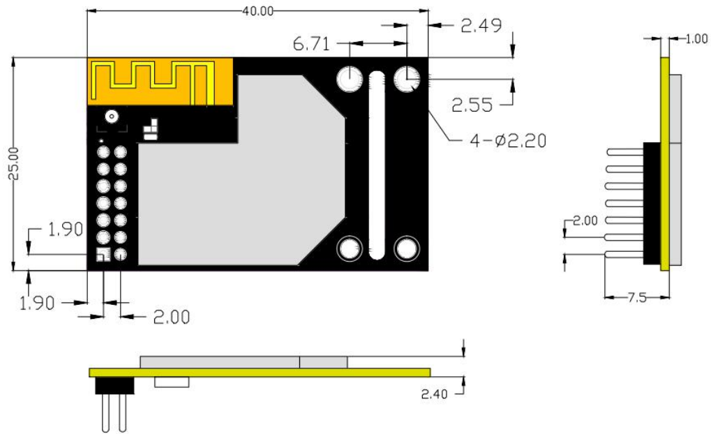
图 7 USR-WIFI232-A2 尺寸图
