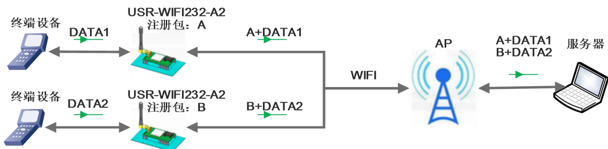
图 27 首次连接发送注册包框图
