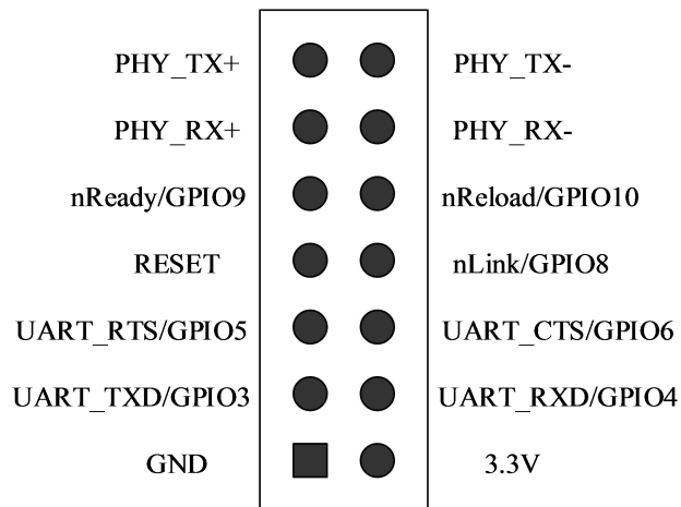
图 6 USR-WIFI232-A2 模块硬件接口定义
