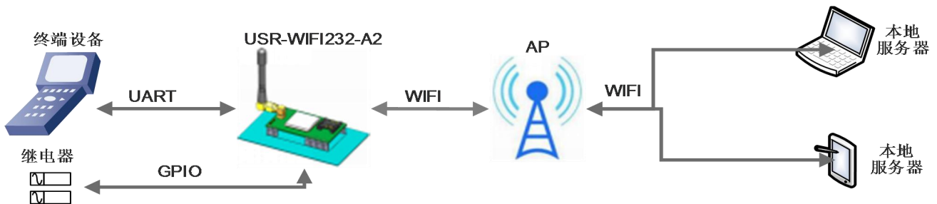
图 18 GPIO 控制框图
