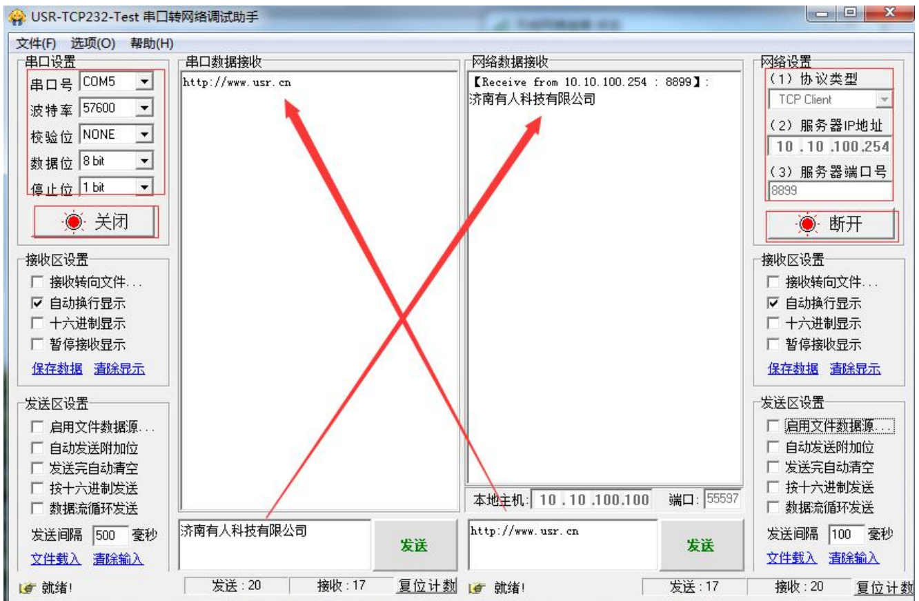
图 4 串口/网络传输测试
