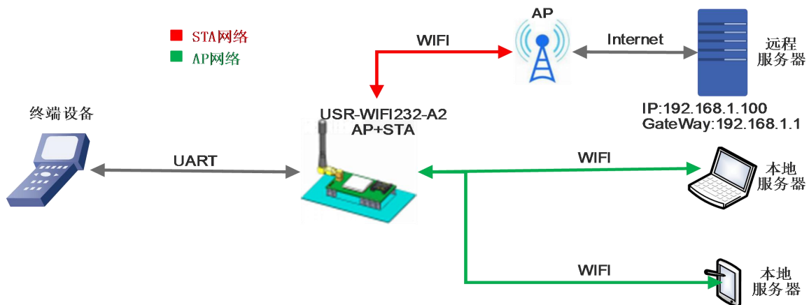
图 13 AP+STA 方式的无线网络
