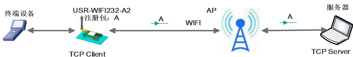
图 27 首次连接发送注册包框图
