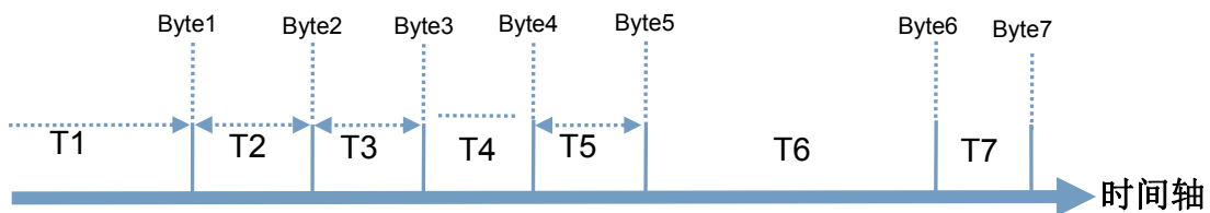
图 23 切换指令模式时序
