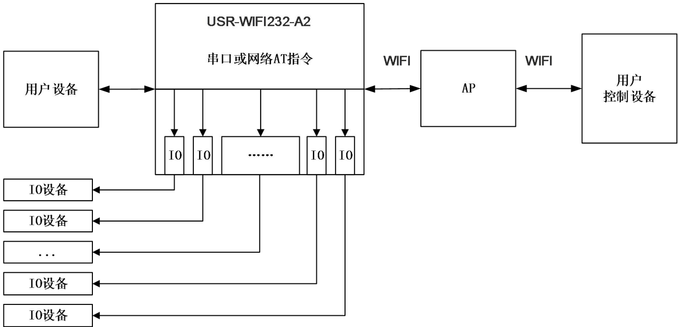
图 17 GPIO 控制框图
