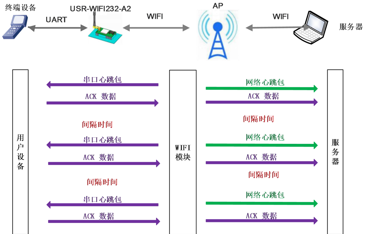
图 34 自定义心跳包框图
