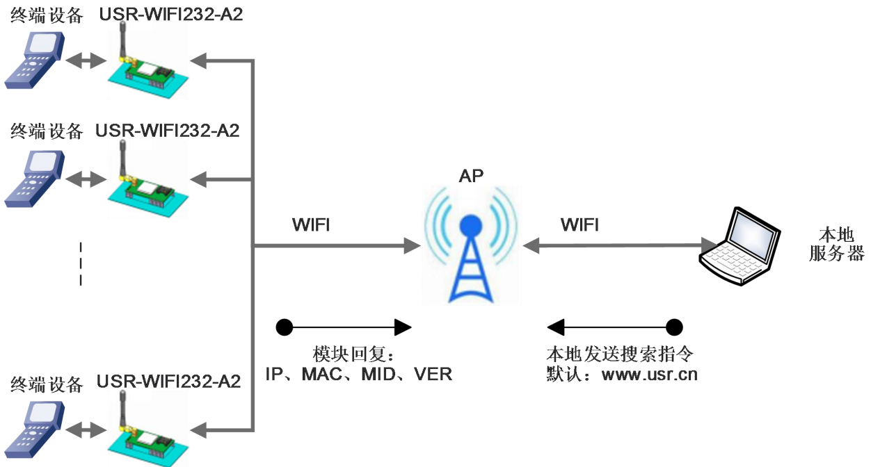
图 33 局域网搜索框图
