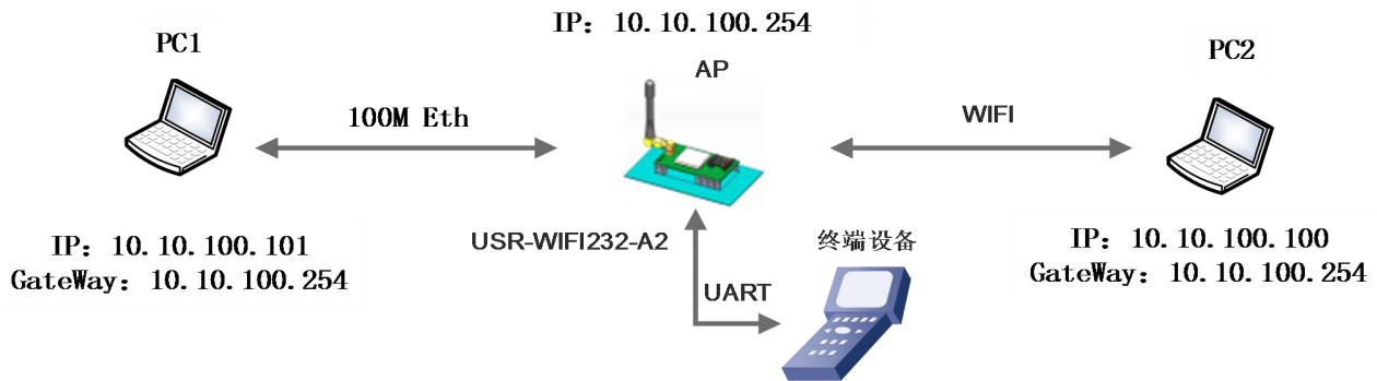
图 15 USR-WIFI232-A2 以太网接口功能（AP LAN）
