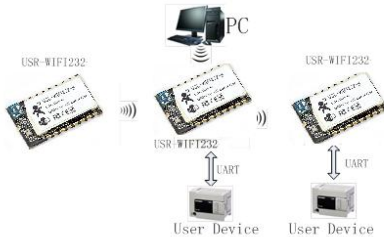
图 3 USR-WIFI232-S 自组网
