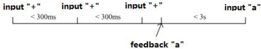
图 9 ‘+++’、‘a’时序要求
