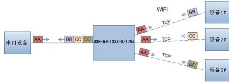
图 4 多 TCP 链接数据传输图示
