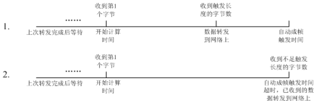
图 1 自动成帧示意图
