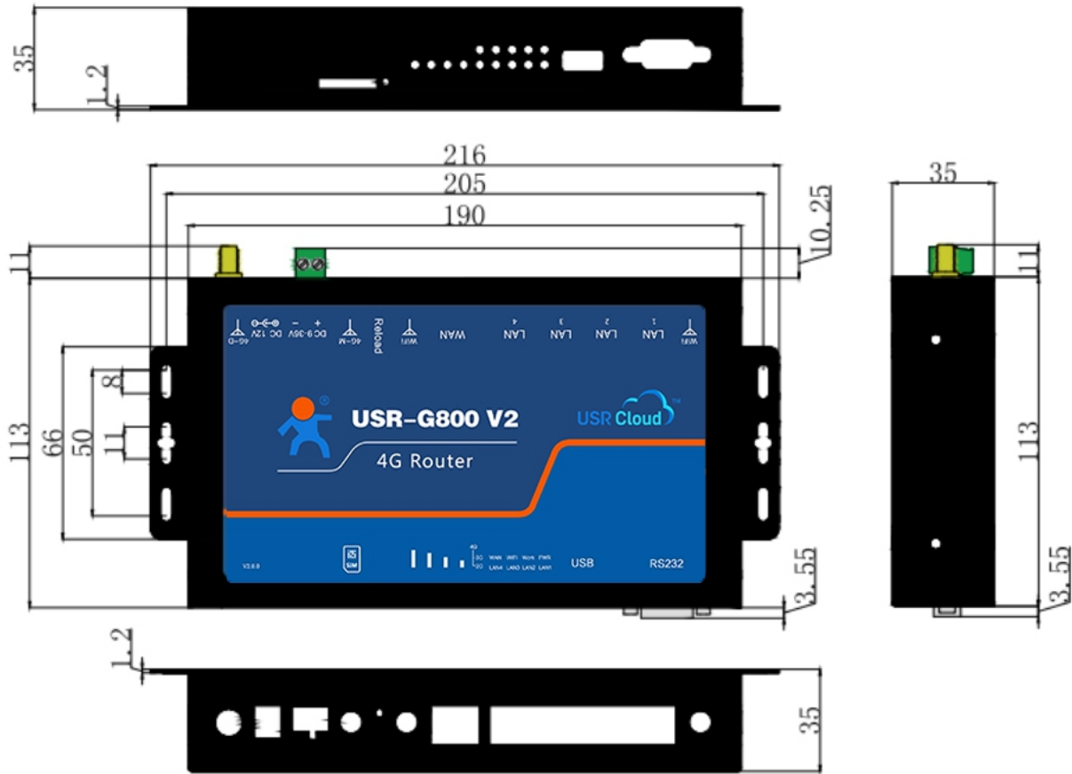
图 1 USR-G800V2 尺寸图
