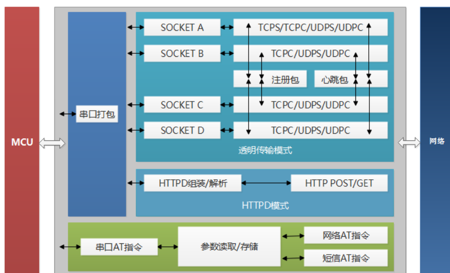
图 32 DTU 功能框图
