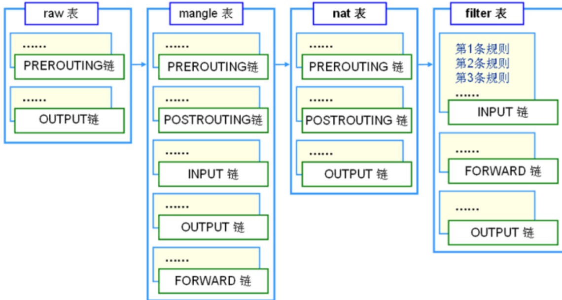
图 24 Linux 系统 iptables 概念框图
