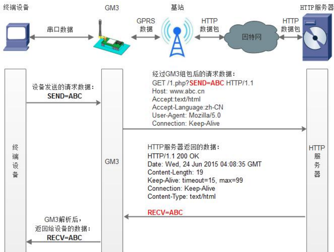
图 10 HTTPD 模式
