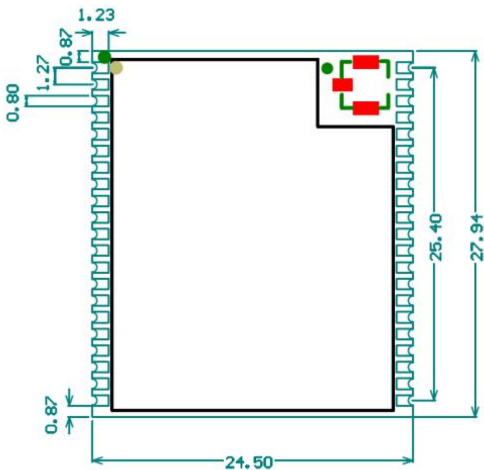
图 6 尺寸示意图
