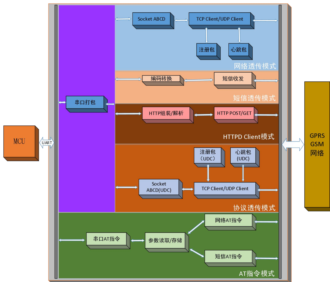
图 7 功能框图
