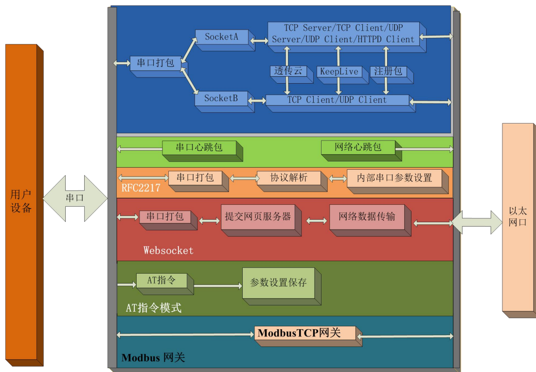
图 1 K3 功能框图
