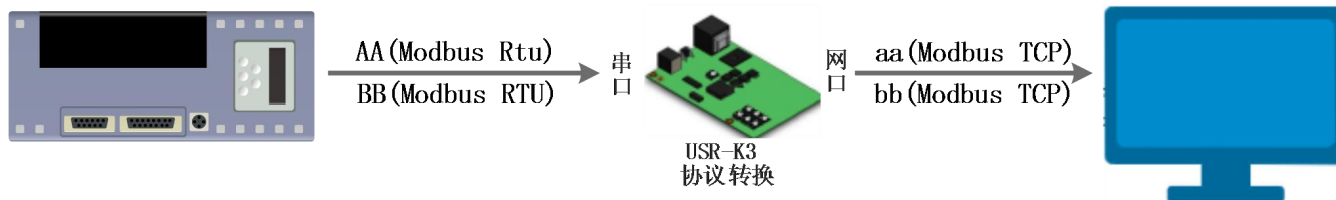
图 36 Modbus TCP
