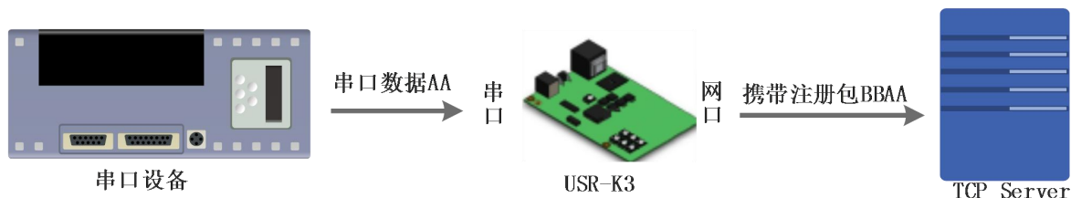
图 49 数据携带注册包
