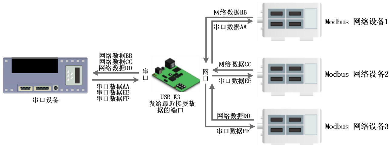
图 43 Modbus TCP
