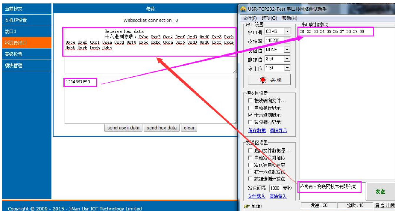
图 28 网页转串口收发数据展示
