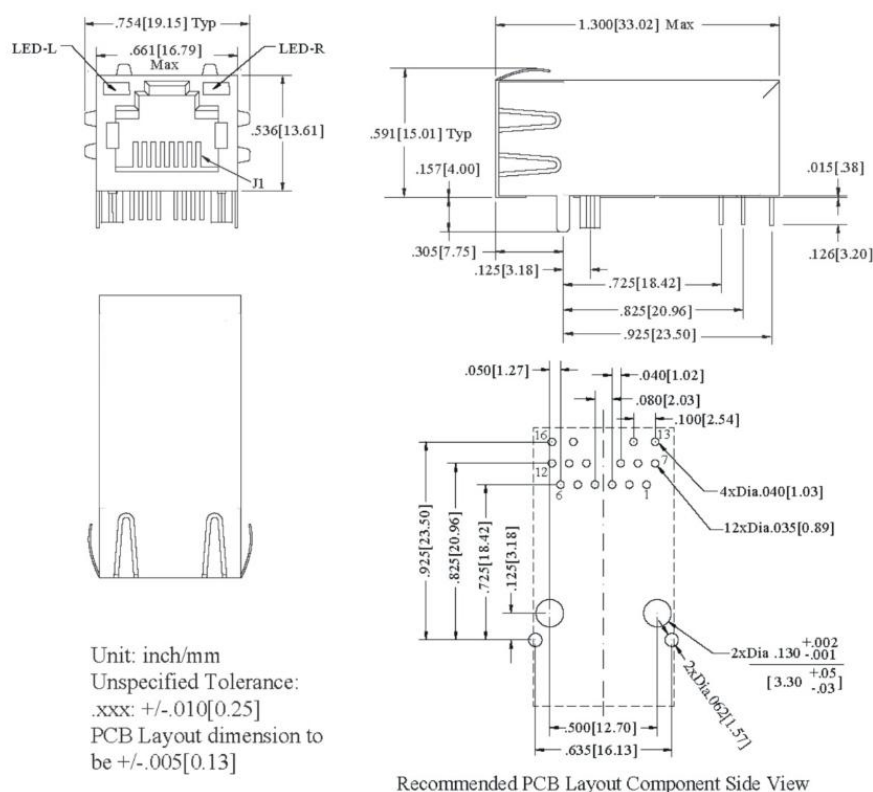
图 8 尺寸图
