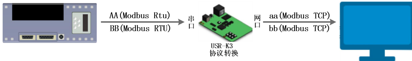
图 30 Modbus TCP
