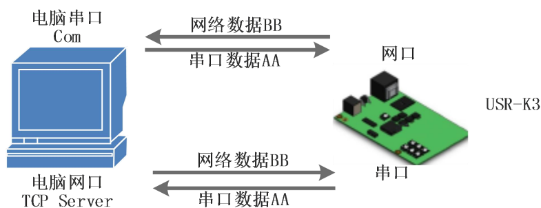
图 3 数据流向
