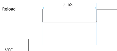
图 21 恢复出厂设置时序图
