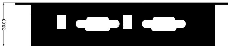
图 9 N540 尺寸图-后侧挡板
