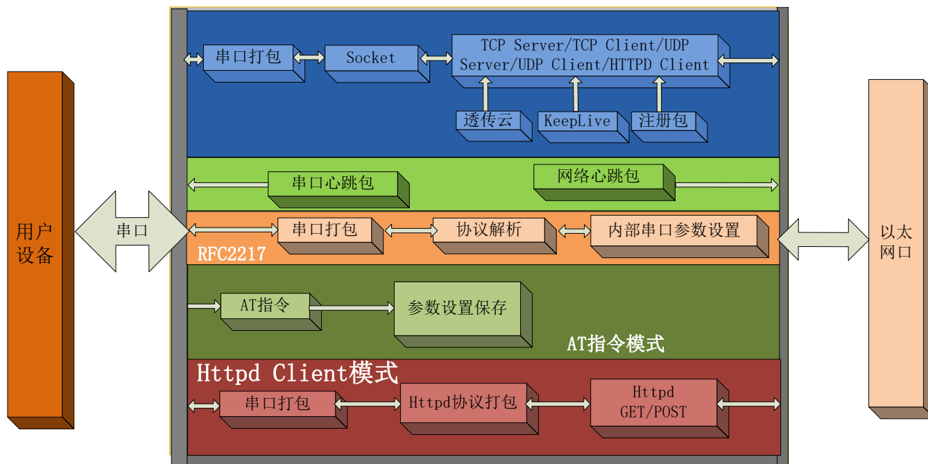
302 功能框图
