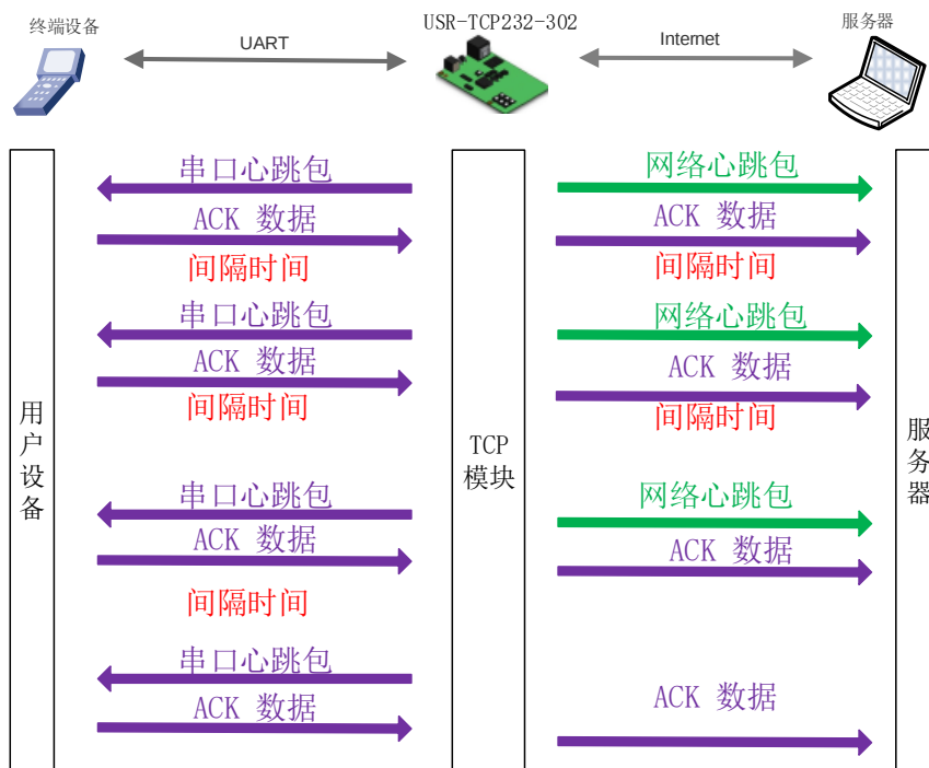
心跳包功能示意图
