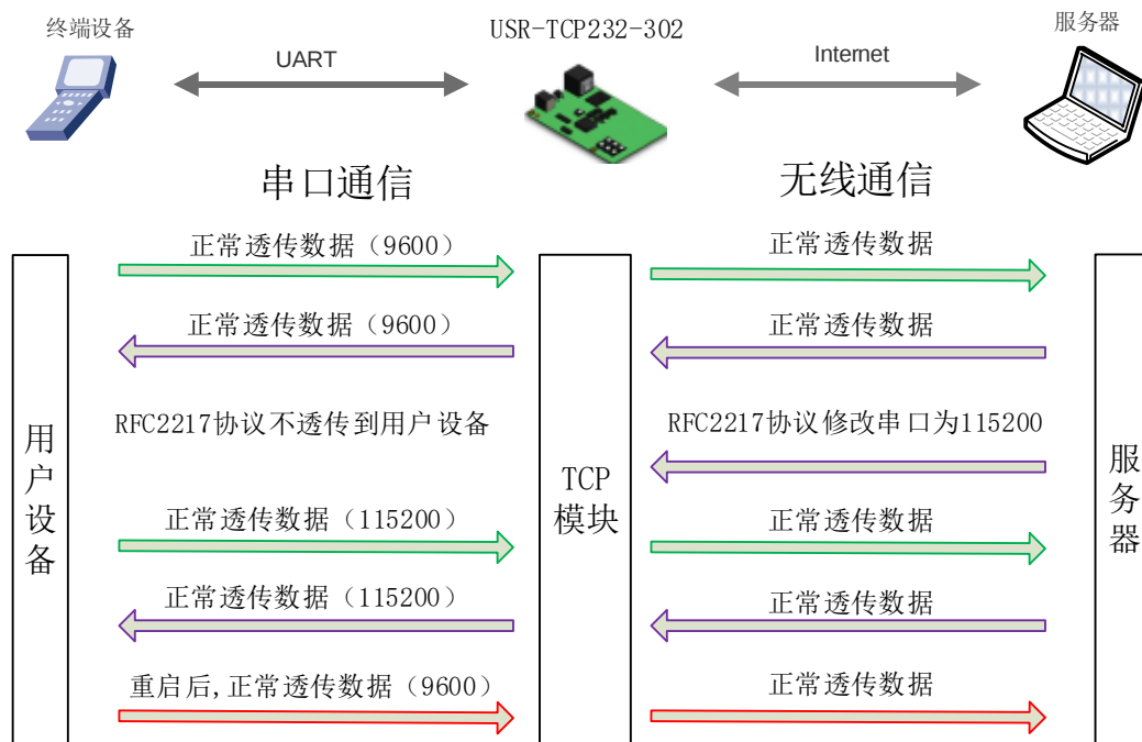
RFC2217 功能框图
