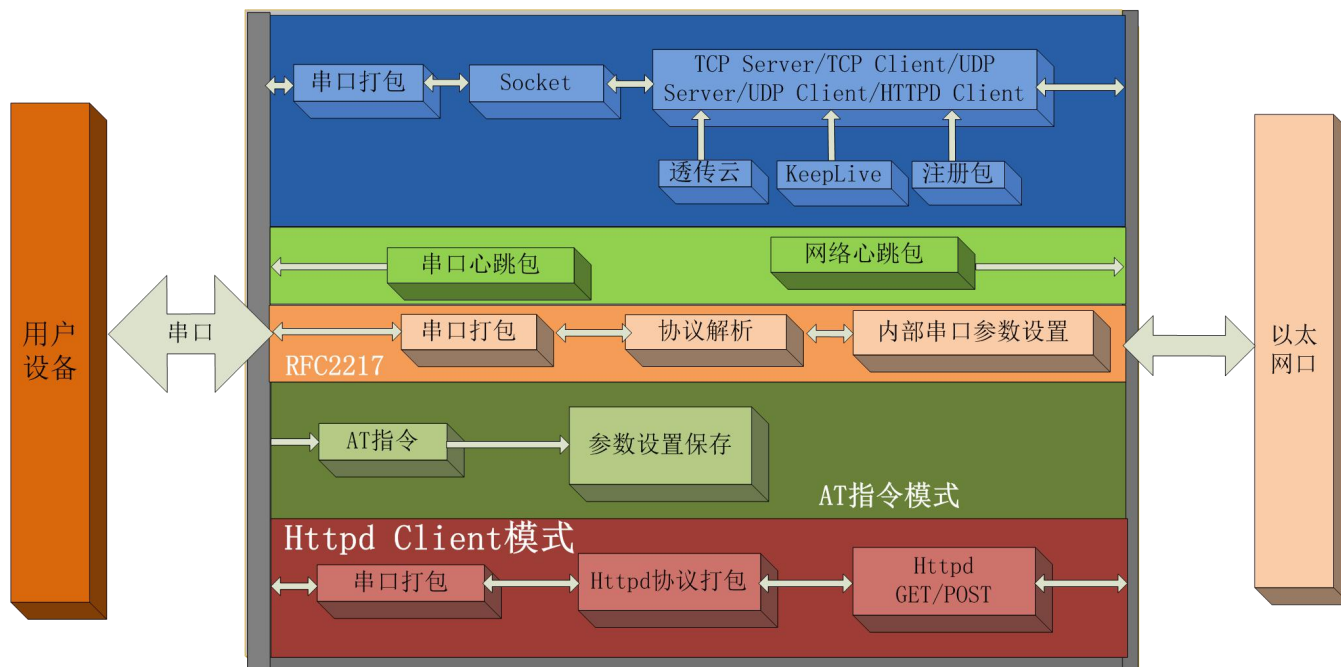
图 1. 306 功能框图
