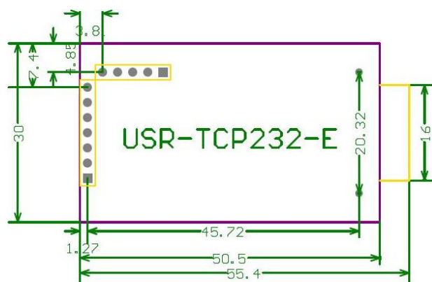
图 7 尺寸图
