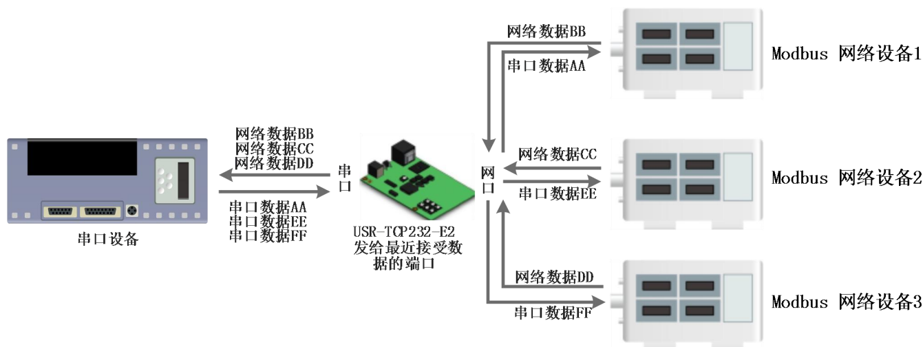
图 30 Modbus TCP 轮询
