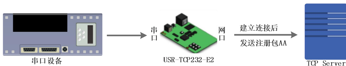
图 31 建立连接发送注册包
