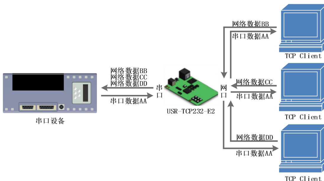
图 15 TCP Server 模式说明
