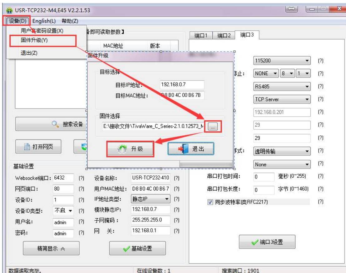
图 44 固件升级
