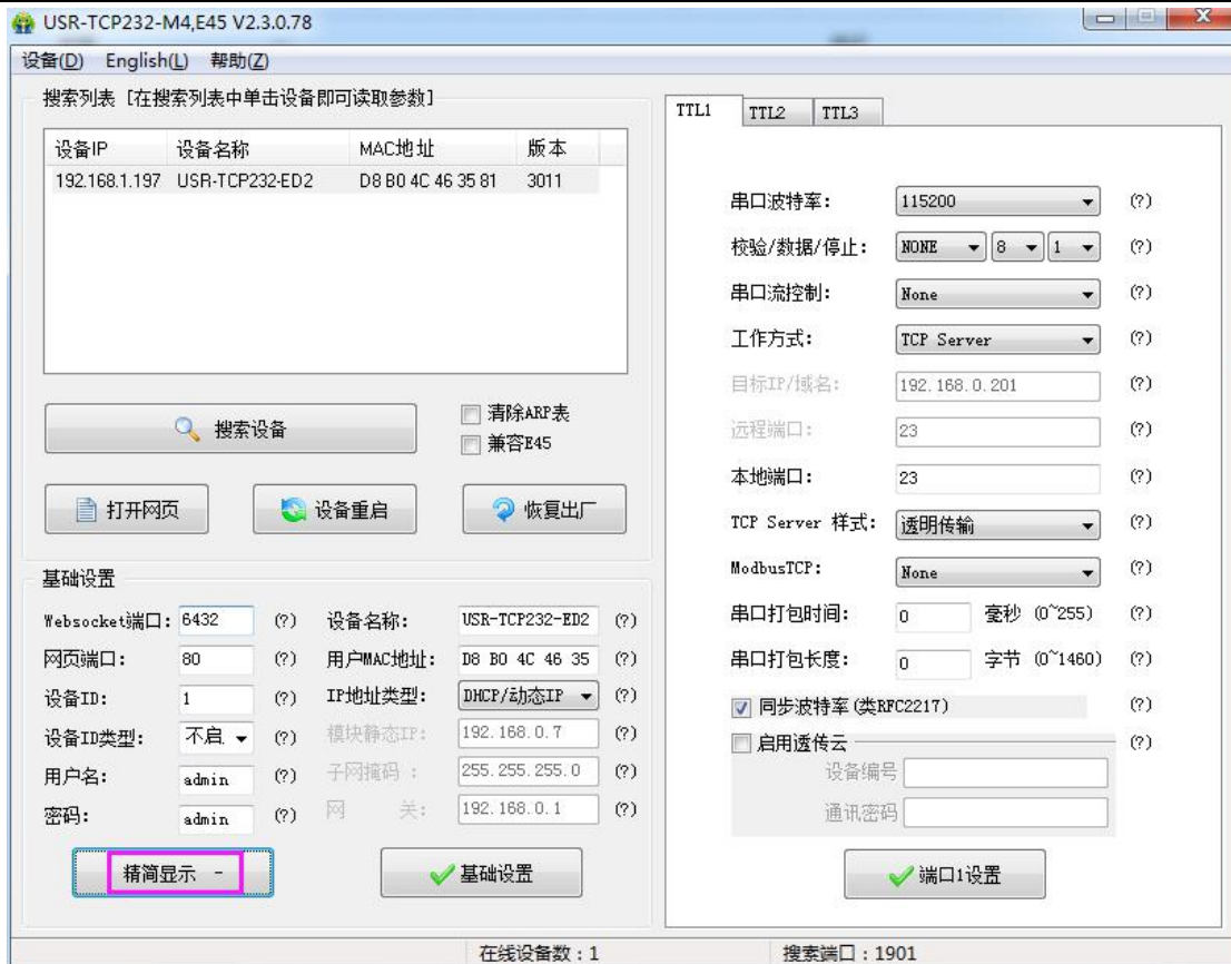
图 41 软件设置参数—完整显示
