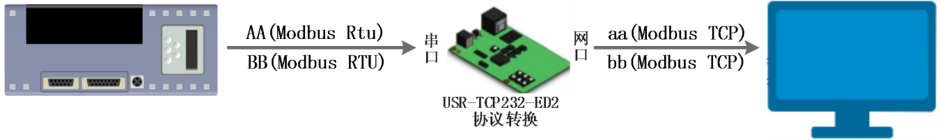
图 29 Modbus TCP
