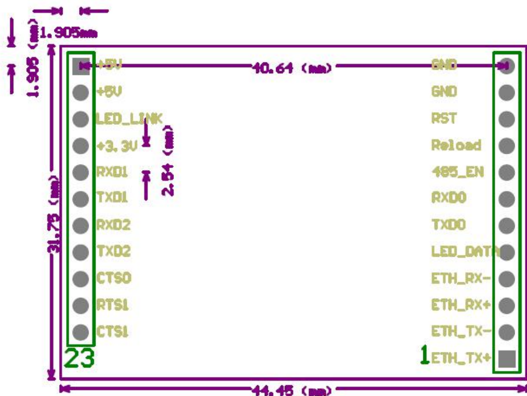
图 7 尺寸图
