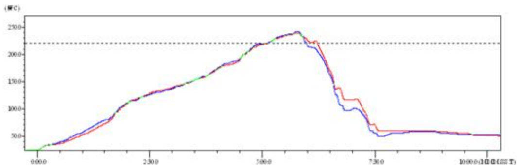
图 11 回流焊焊接温度曲线图
