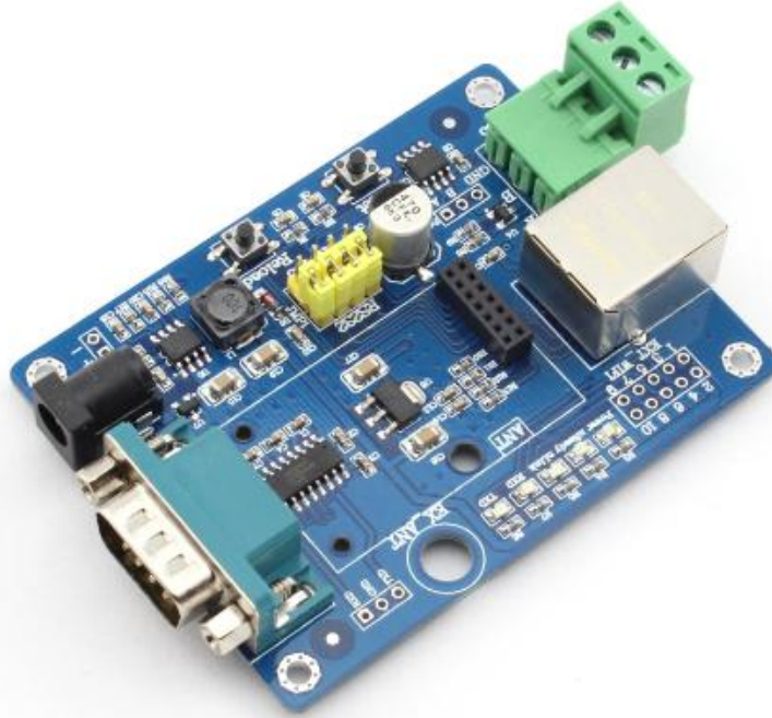
图 3 USR-WIFI232-A2 模块评估板
