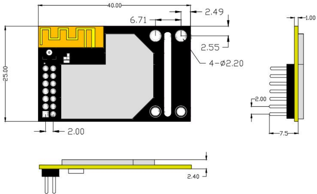
图 2 USR-WIFI232-A2 尺寸图
