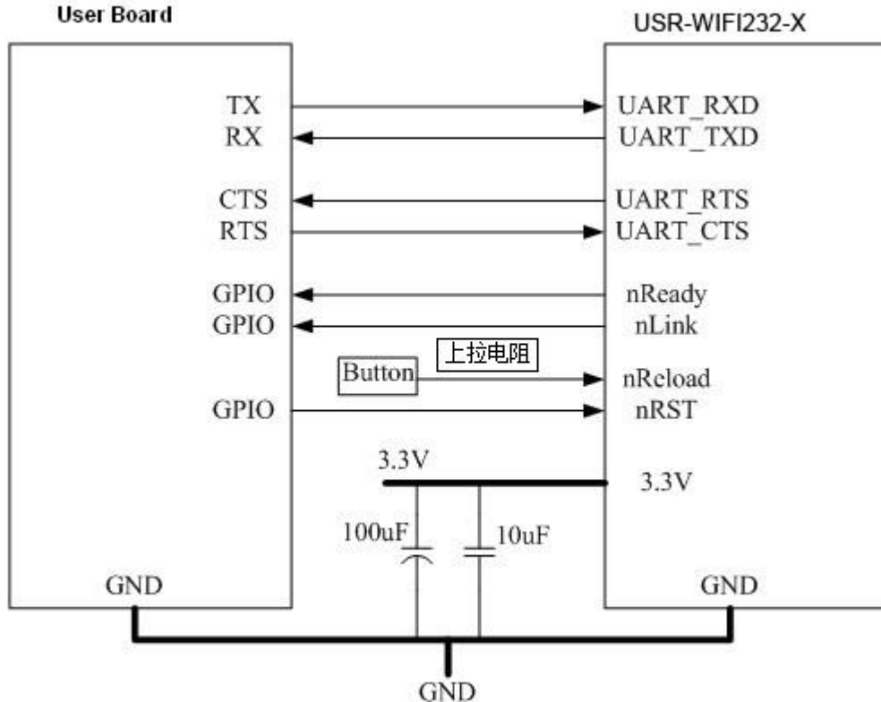
图 4 USR-WIFI232-A2 典型应用硬件连接
