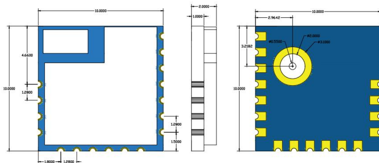
图 8. WH-BLE103 尺寸示意图
