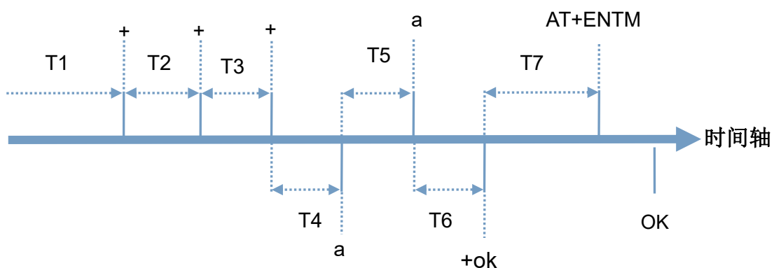
图 25. +++a 时序图
