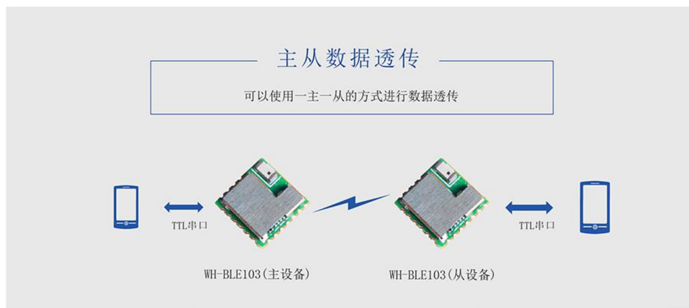
图 13. 主从数据透传示意图
