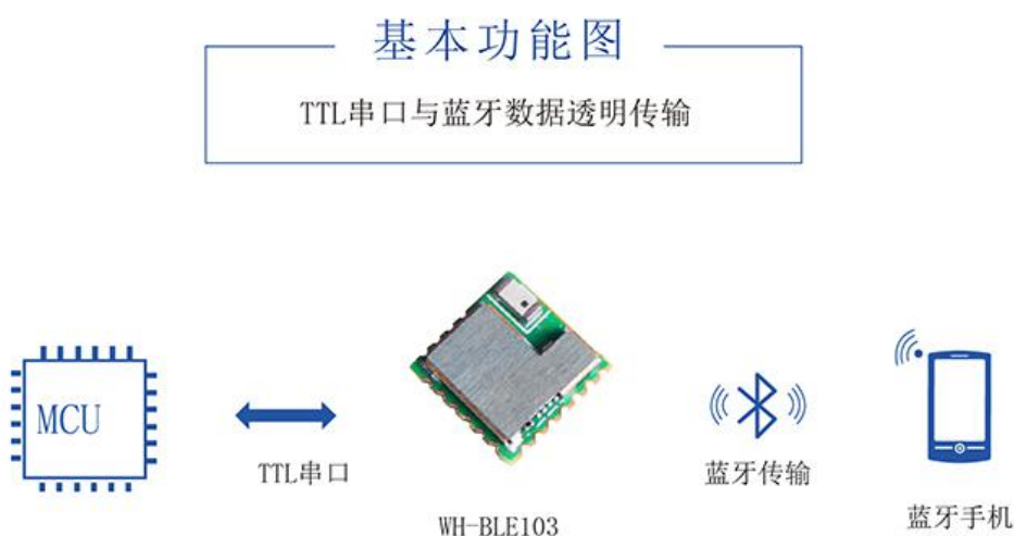
图 7. 模块基本功能传输图
