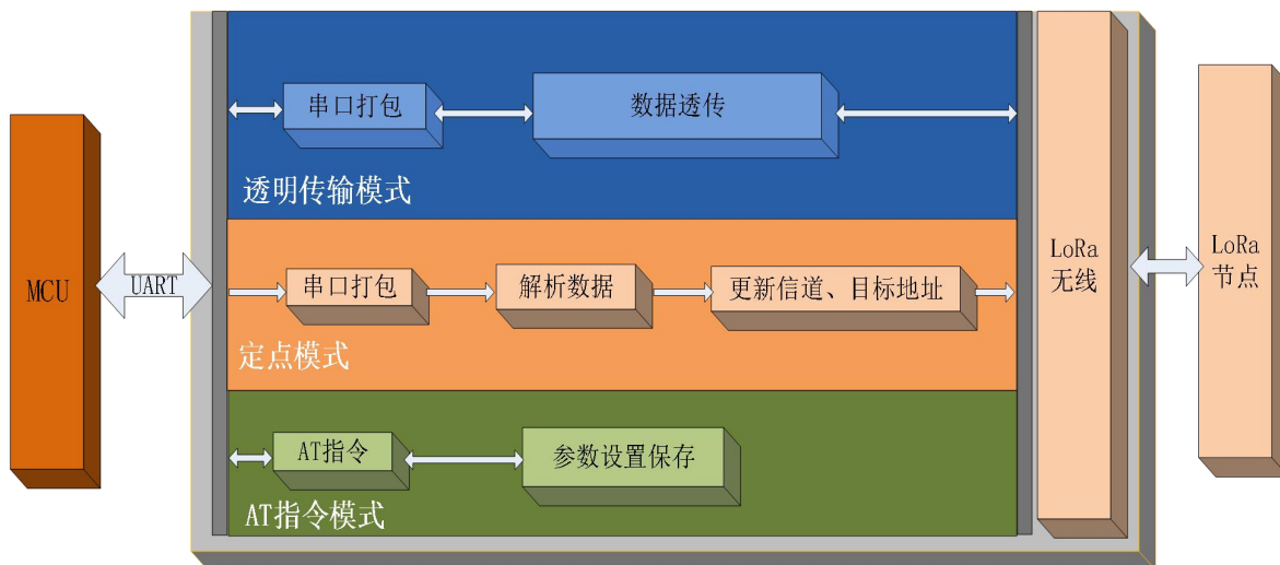
图 5 功能框图
