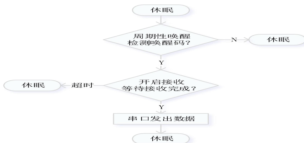
图 8 WU 和 LR 模式工作流程
