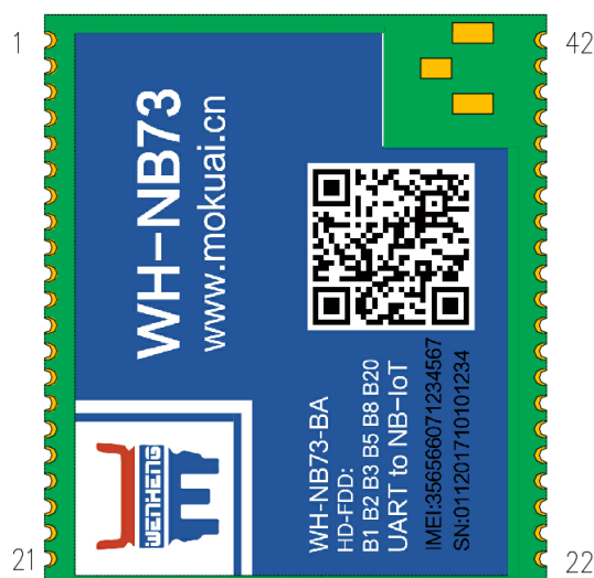
图片4 WH-NB73-BA 引脚标号
