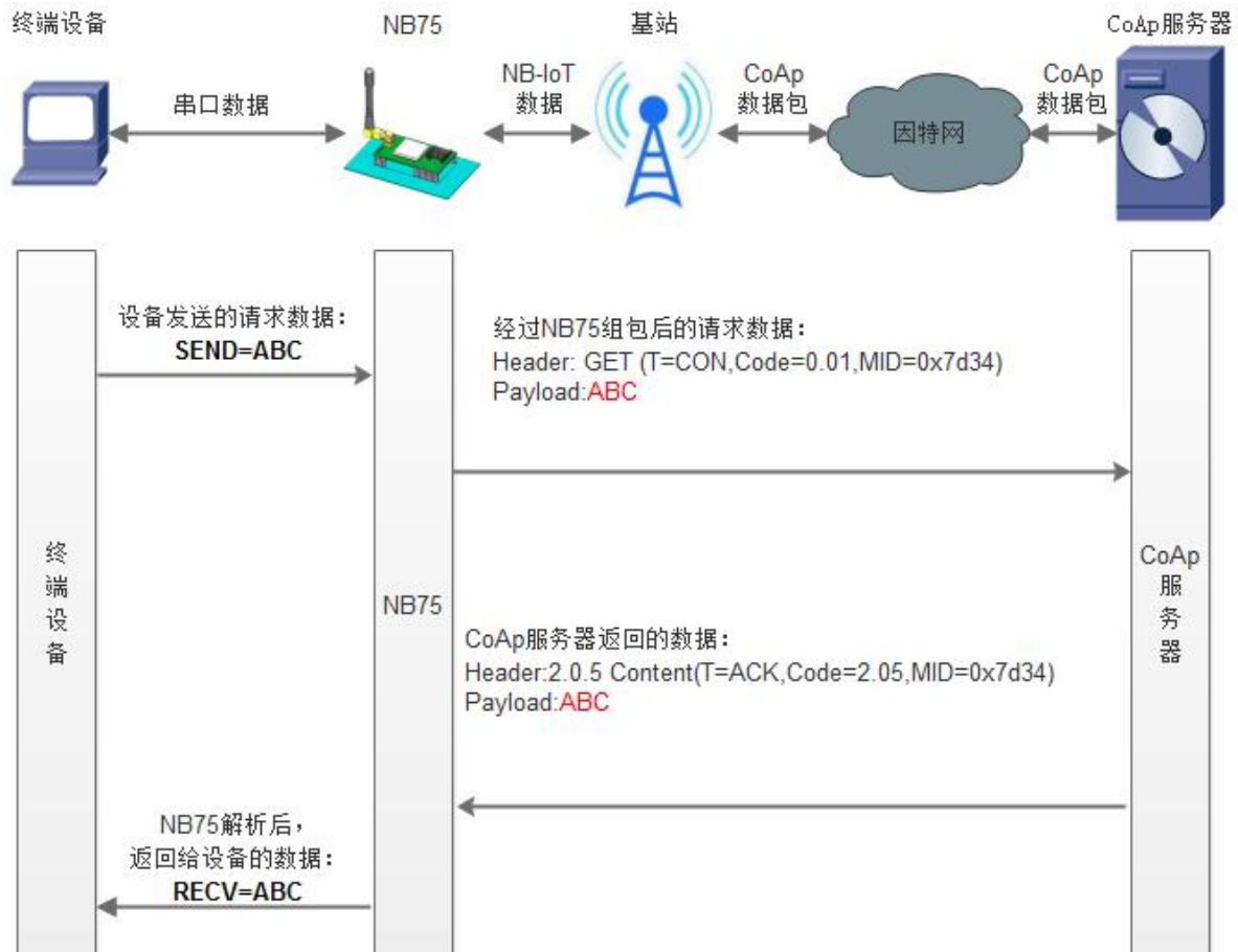
图 8 CoAP 模式
