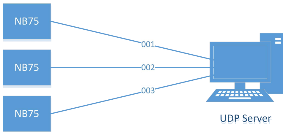
图 13 注册包功能示意图
