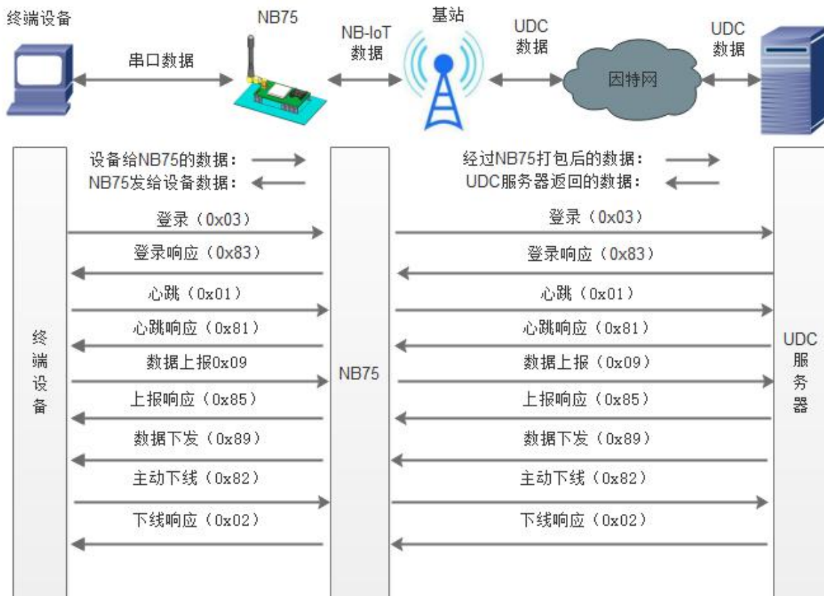
图 9 协议透传模式
