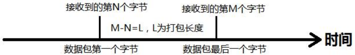
图 11 长度触发模式
