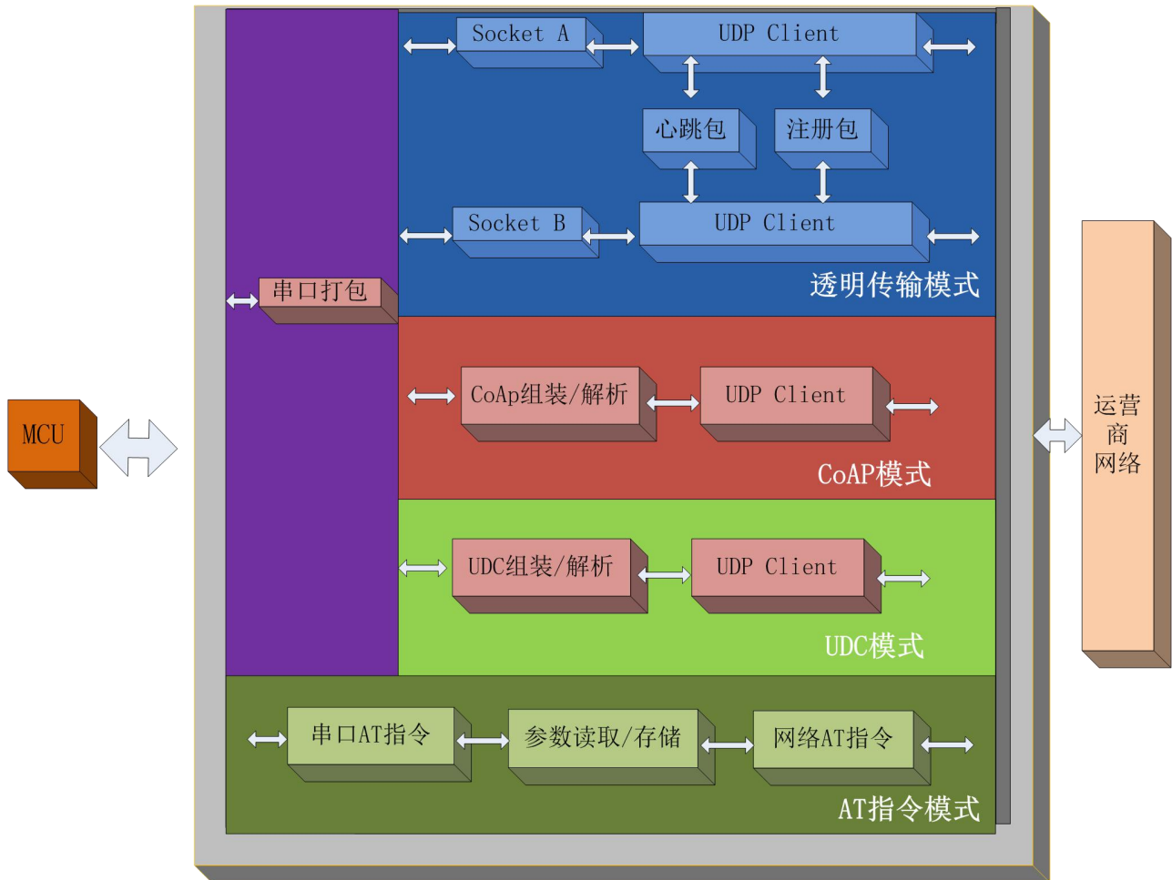
图 6 功能框图
