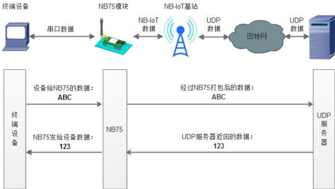
图 7 网络透传模式
