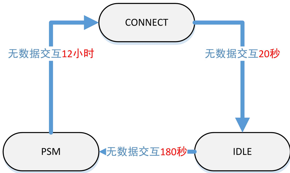
图 12 网络连接状态切换示意图
