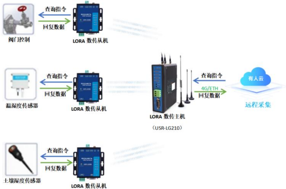
图 3 智慧农业系统示意图
