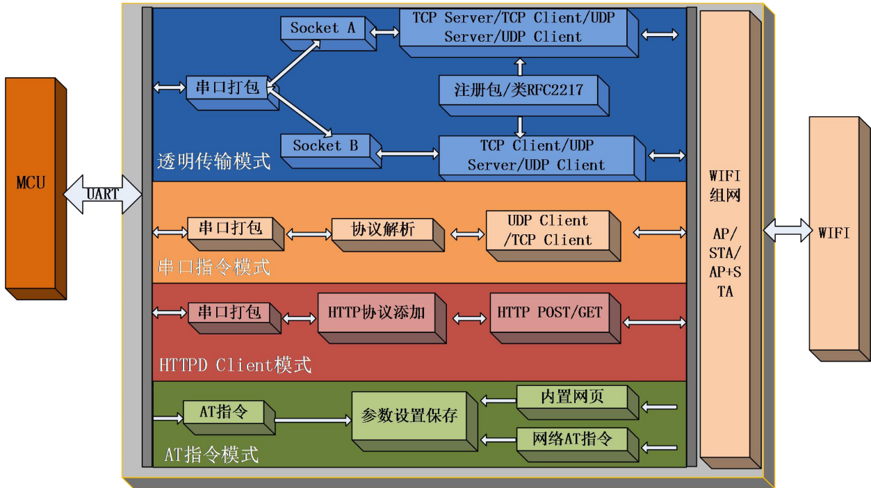
图 2 功能框图
