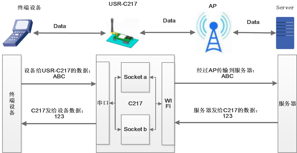
图 6 AP+STA 模式组网
