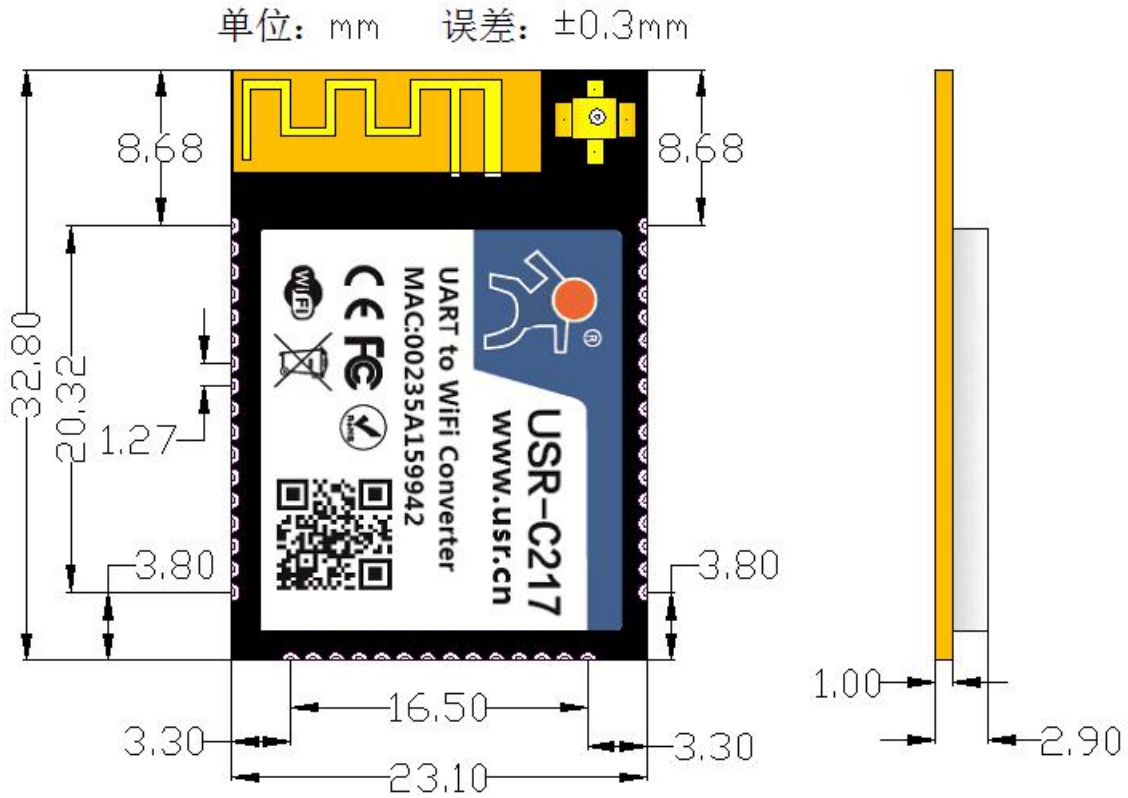
图 7 USR-C217 尺寸图
