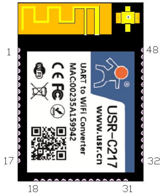
图 8 USR-C217 引脚图
