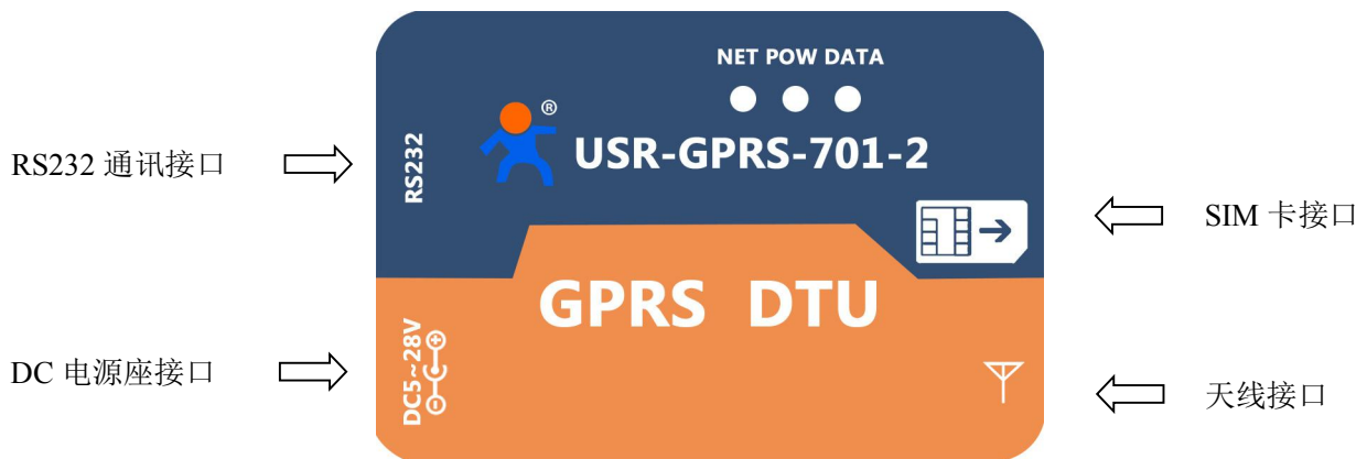
图 1 USR-GPRS232-701-2 接口图
