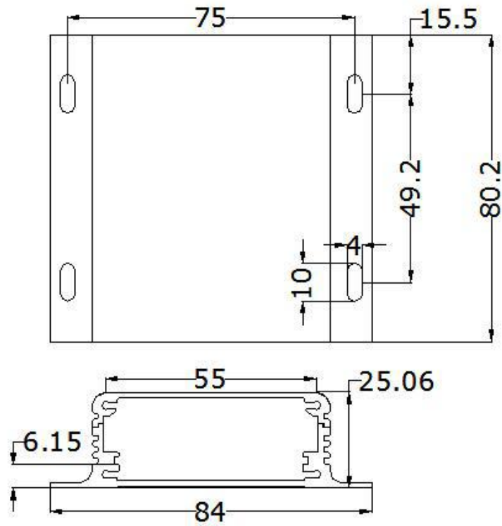
图2 USR-GPRS232-701-2 尺寸图
