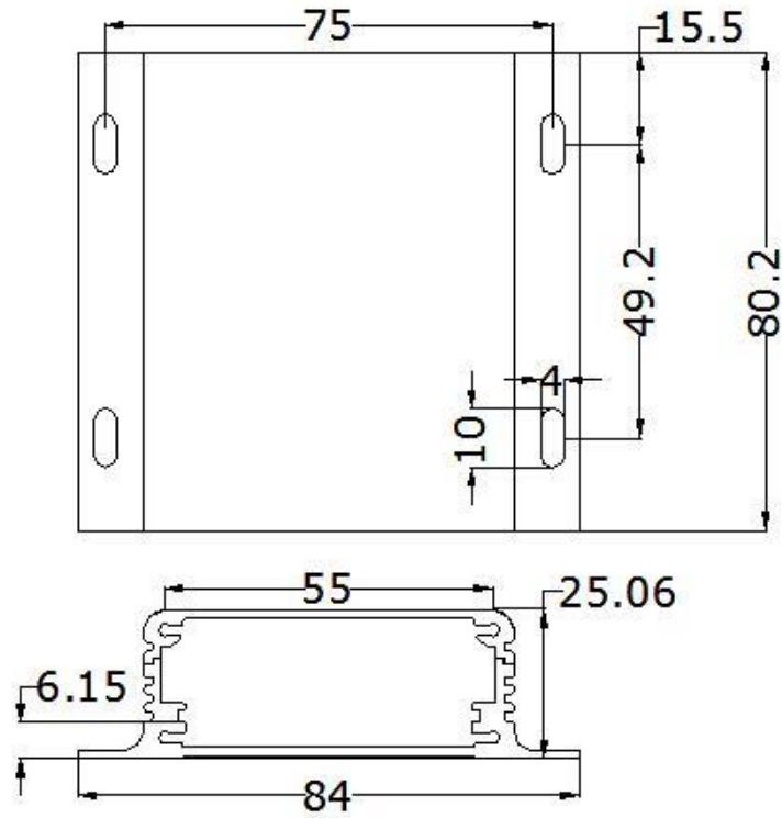
图 2 USR-GPRS232-720 尺寸图
