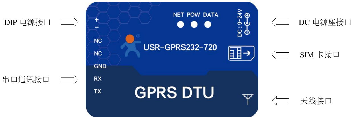
图 1 USR-GPRS232-720 接口图
