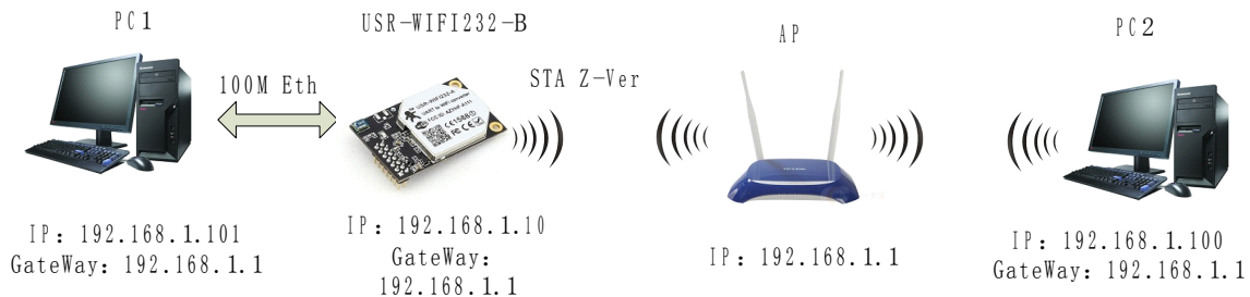
图 7 USR-WIFI232-B 以太网接口功能（STA Z-Ver）
