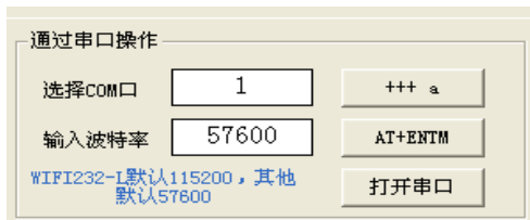
图 23 设置软件串口参数示意图
