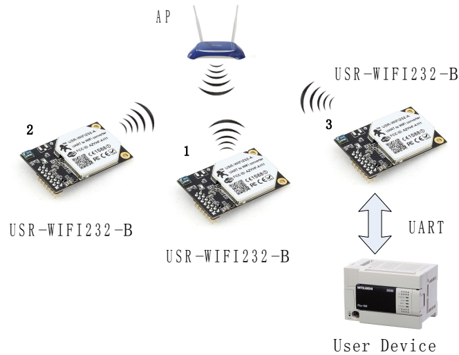
图 2 基于 STA 的无线网络
