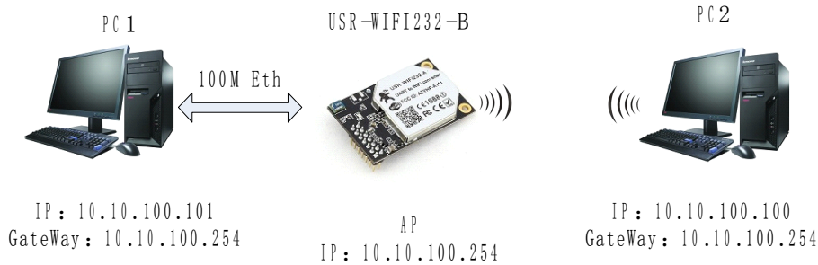
图 5 USR-WIFI232-B 以太网接口功能（AP）
