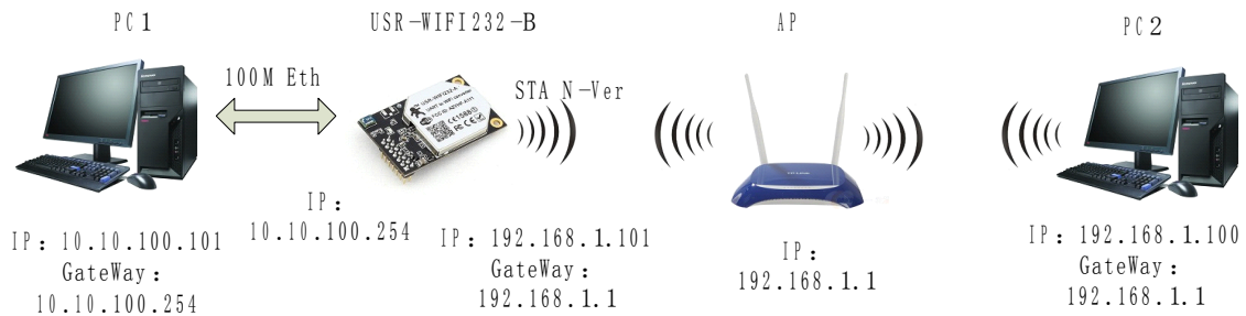
图 6 USR-WIFI232-B 以太网接口功能（STA N-Ver）
