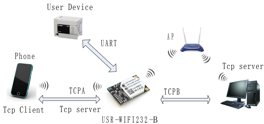
图 4 AP+STA 方式的无线网络
