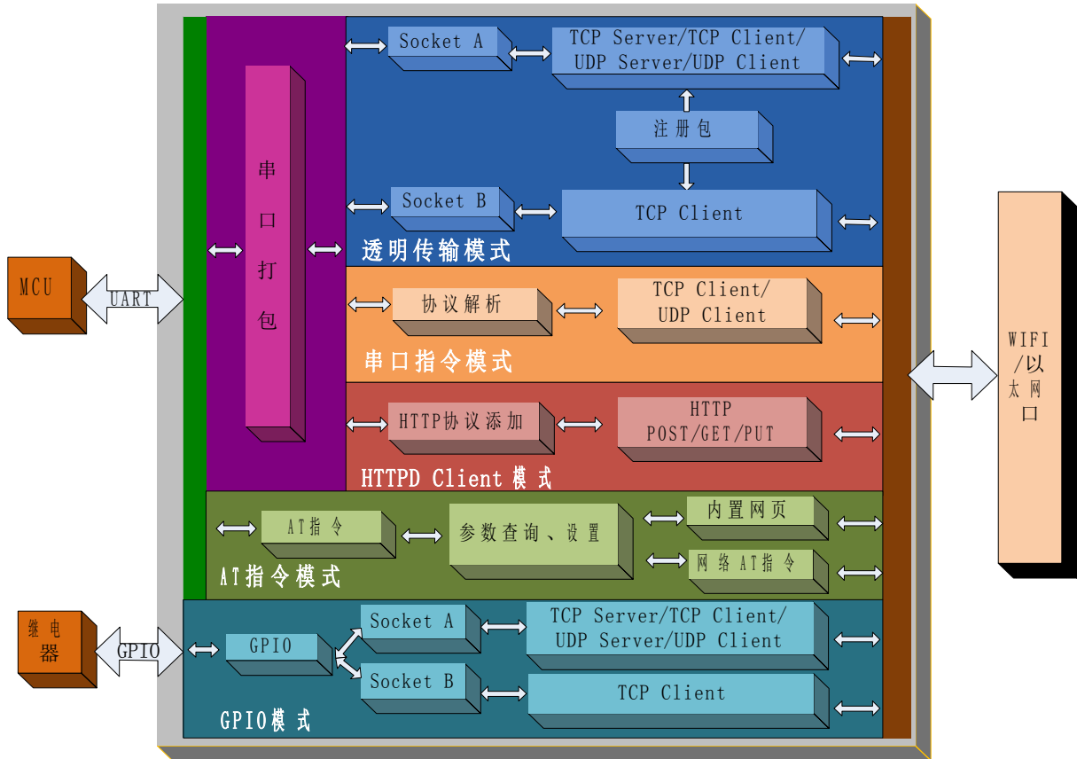
图 1 USR-WIFI232-B 功能框图
