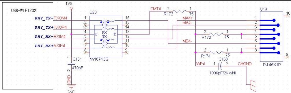
图 7 USR-WIFI232-B 模块带网络变压器的应用
