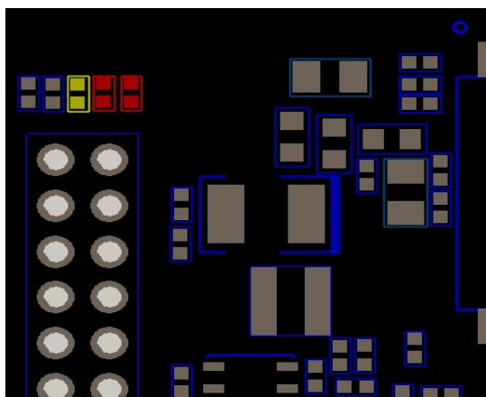
图 9 BOT 层元件图
