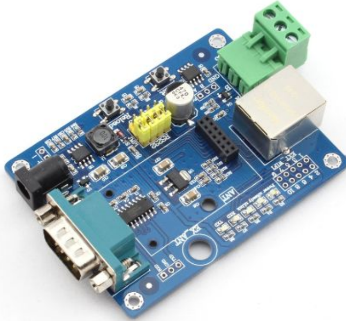
图 3 USR-WIFI232-B 模块评估板
