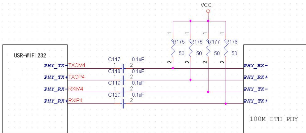
图 8 USR-WIFI232-B 模块不带网络变压器的应用
