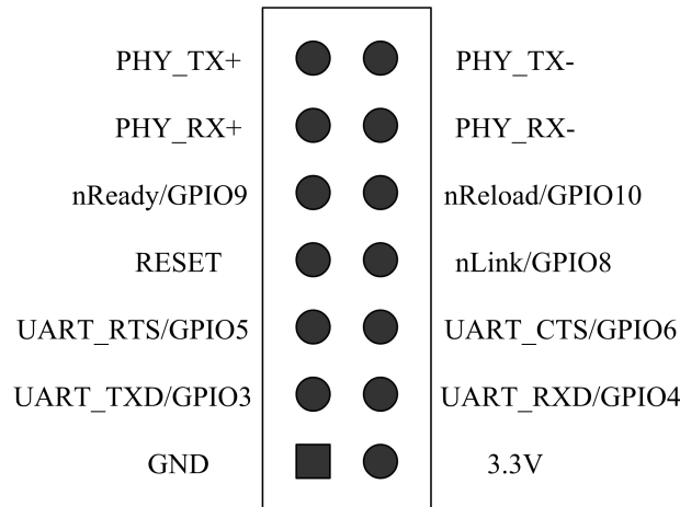
图 1 USR-WIFI232-B 模块接口定义
