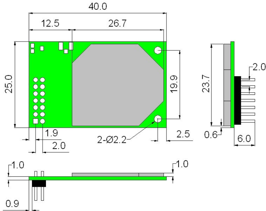
图 2 USR-WIFI232-B 尺寸图
