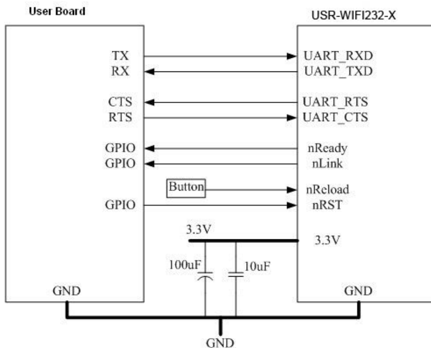
图 4 USR-WIFI232-B 典型应用硬件连接
