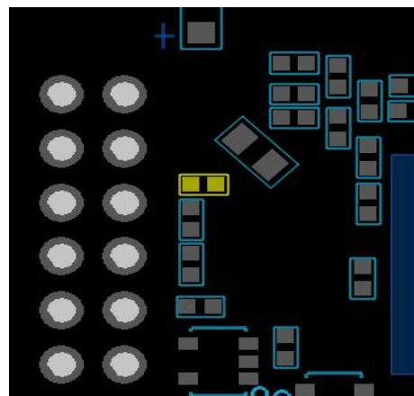
TOP 层元件图
