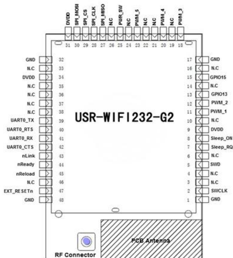
图 8 USR-WIFI232-G2 引脚图
