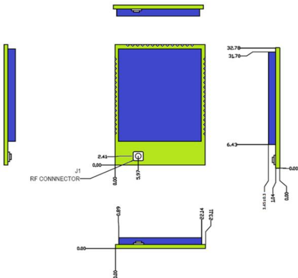
图 9 USR-WiFi232-G2 尺寸图(单位: mm)
