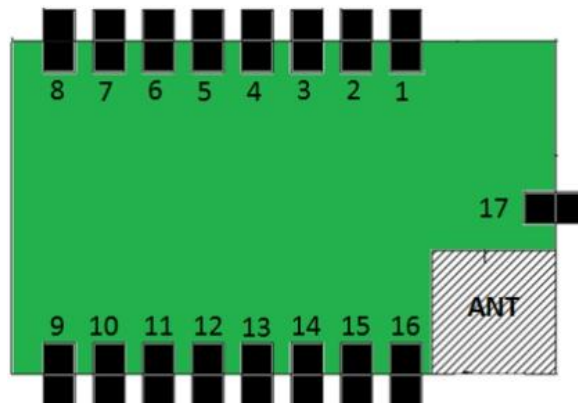
图 1 USR-WIFI232-S 引脚图
