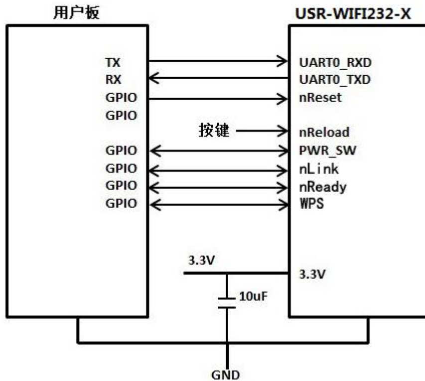
图 5 USR-WIFI232-S UART 应用硬件连接
