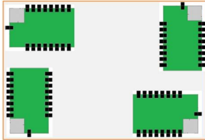
Figure 1 USR-WIFI232-Sa 模组建议放置区域
