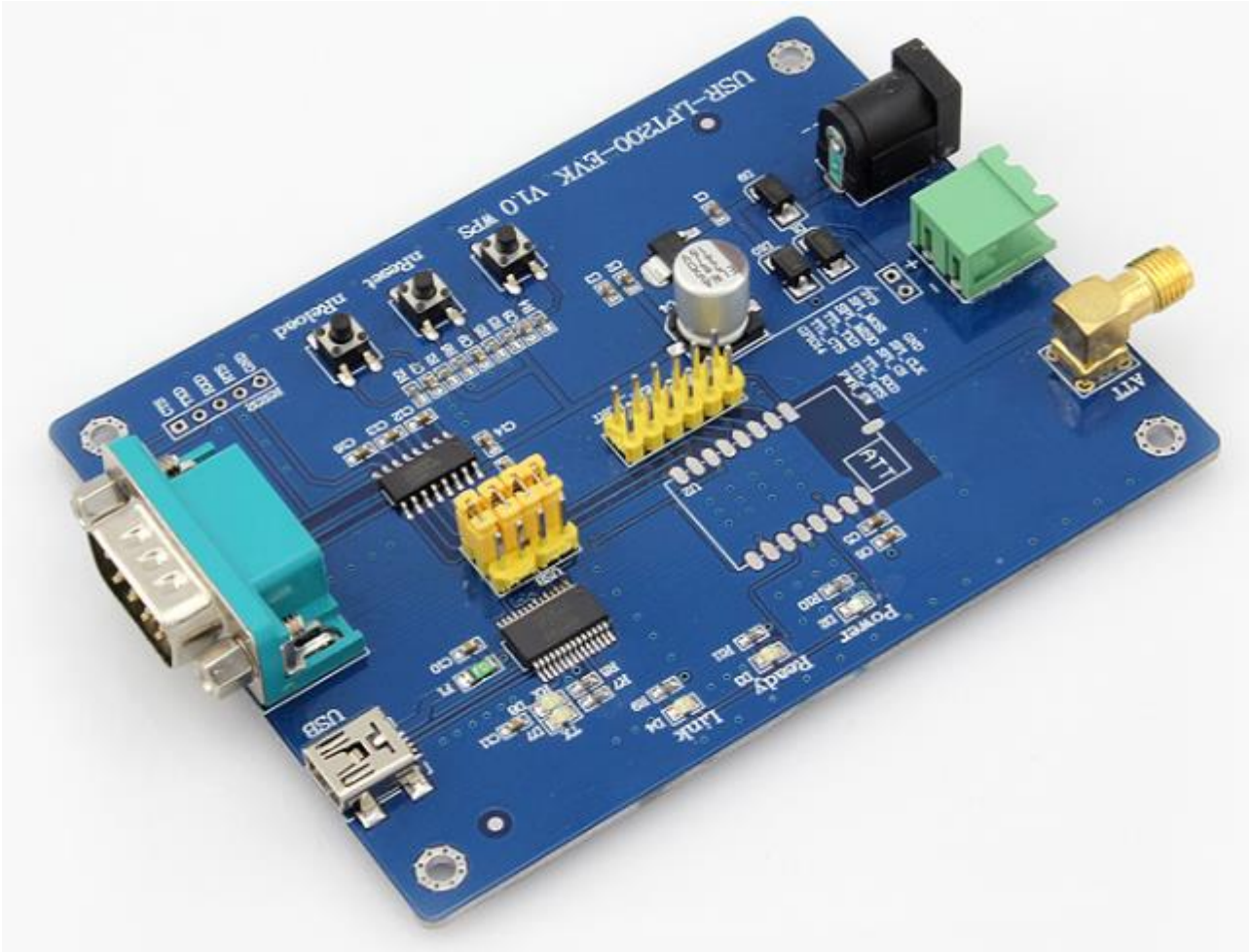
图 4 USR-WIFI232-S 模块评估板 USR-WIFI232-S 模块评估板接口描述
