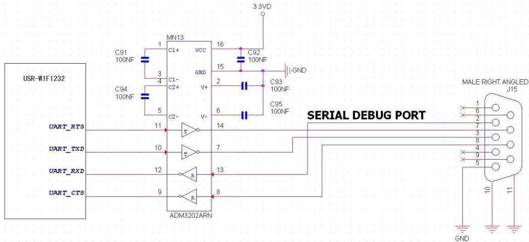
图 6 UART 接口参考设计
