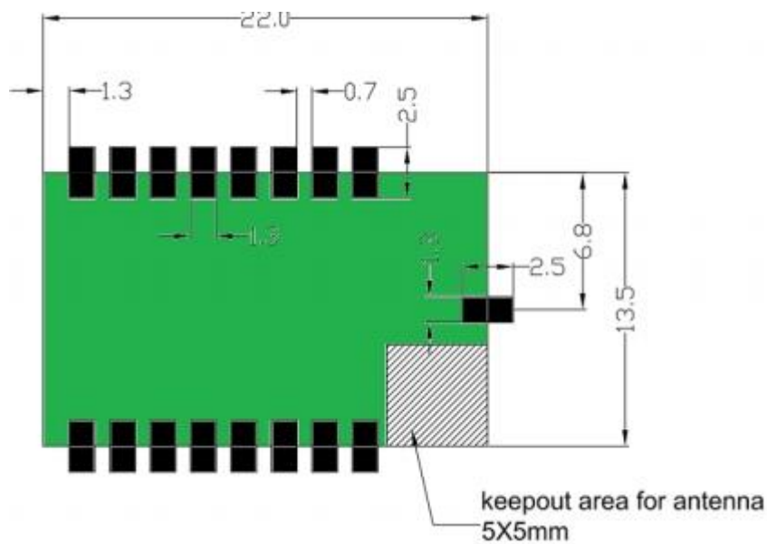
图 3 USR-WIFI232-S PCB 尺寸图 (单位:mm)
