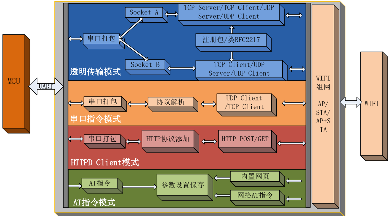
图 2 功能框图
