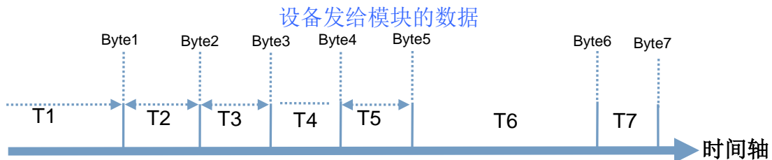
图 14 成帧机制
