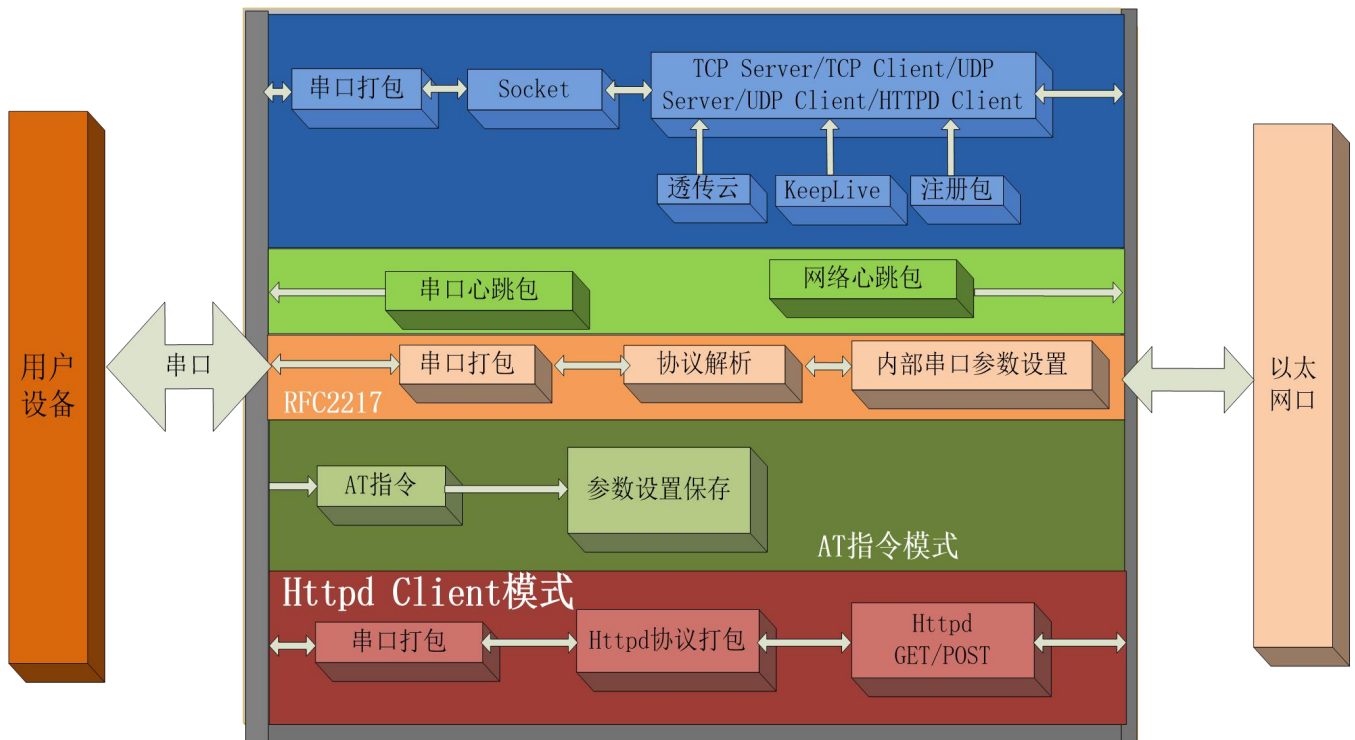
图 1 302 功能框图
