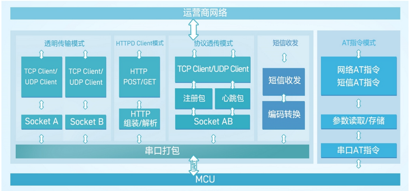
图 3. 功能框图
