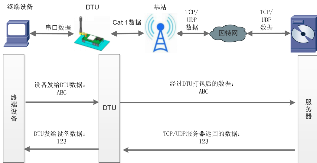
图 4. 网络透传模式
