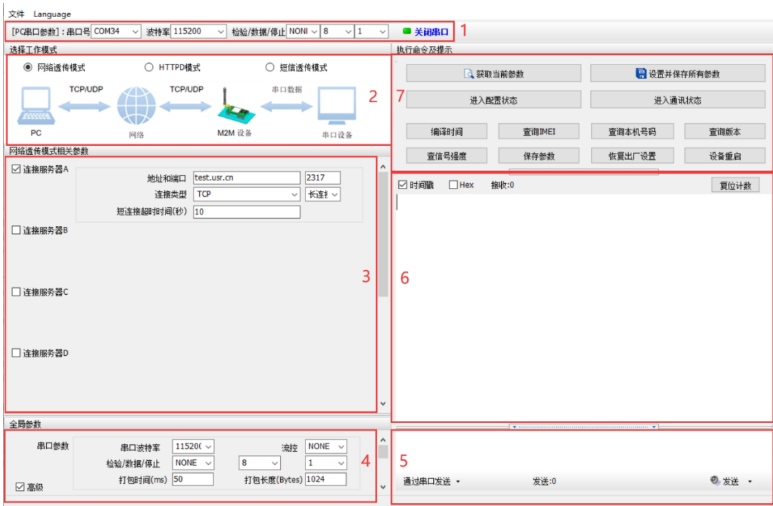
图 22. 设置软件示意图
