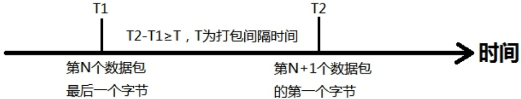
图 23. 时间触发模式
