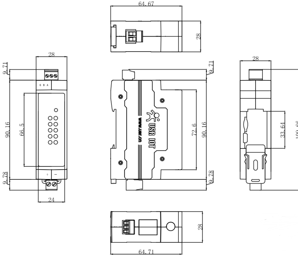
图 2. USR-DR502/DR512 尺寸图
