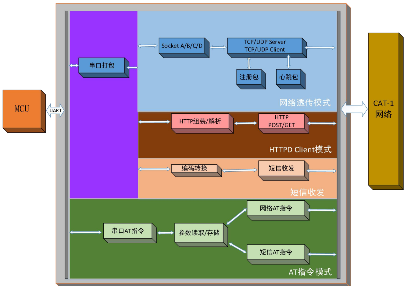
图 4. 功能框图
