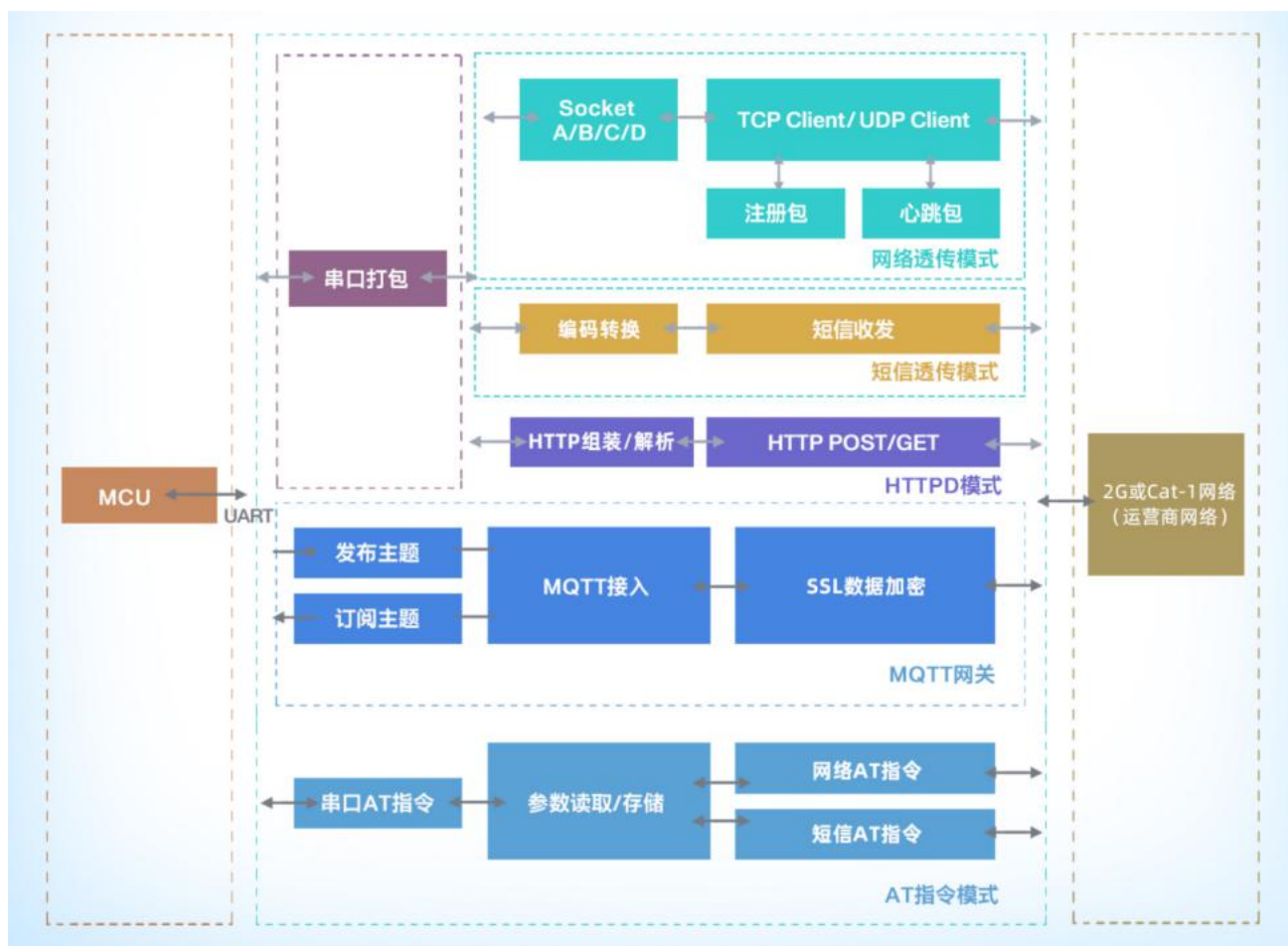
图 1. 功能框图
