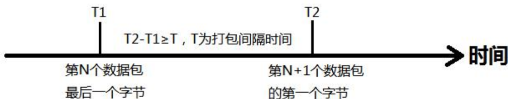
图 30. 时间触发模式
