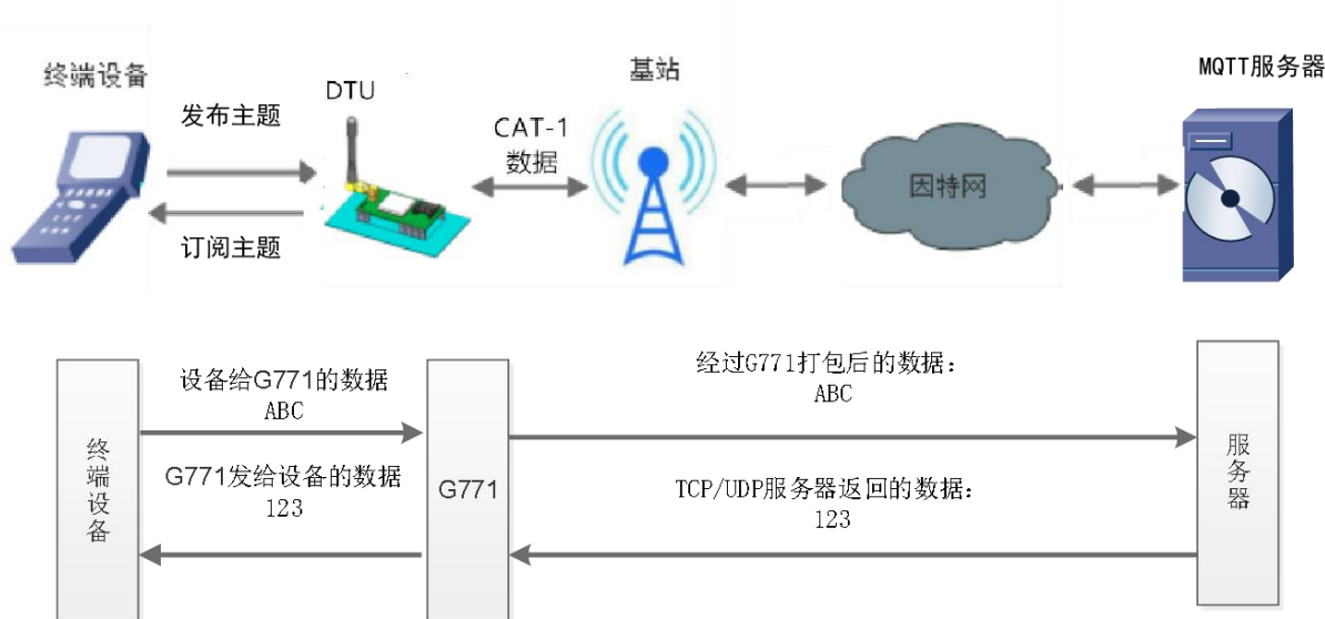
图 15. MQTT 模式
