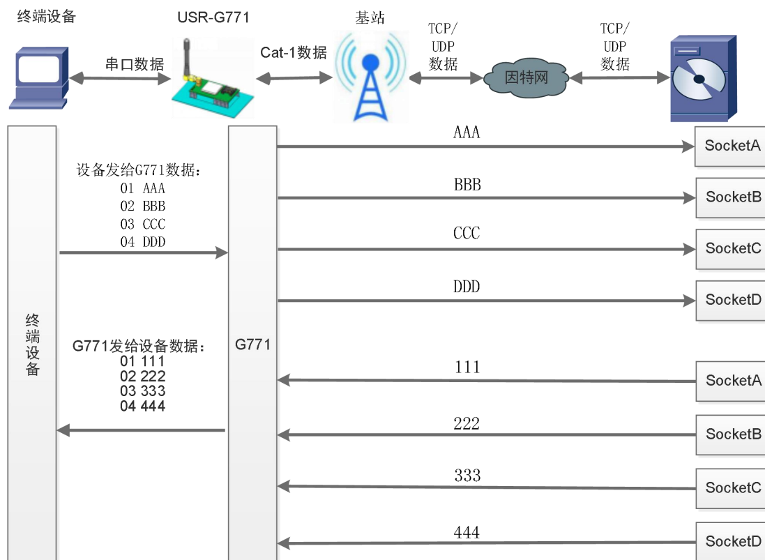
图 27. 套接字分发协议示意图
