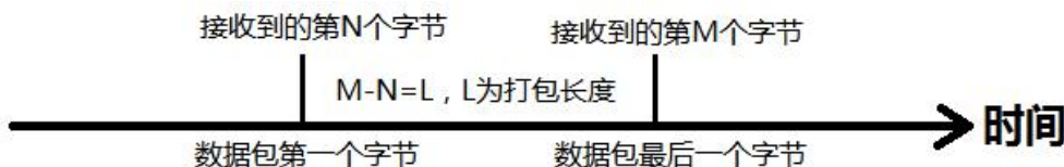
图 31. 长度触发模式
