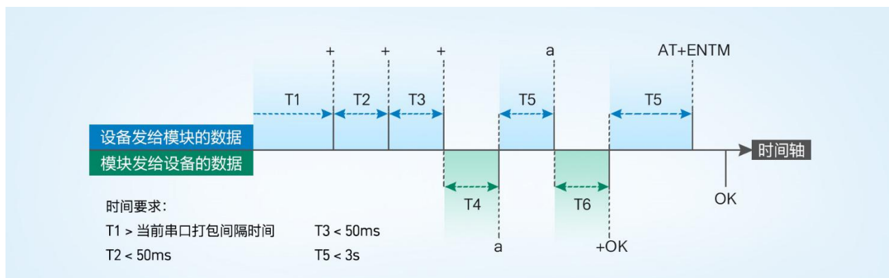
图 32. 切换指令模式时序
