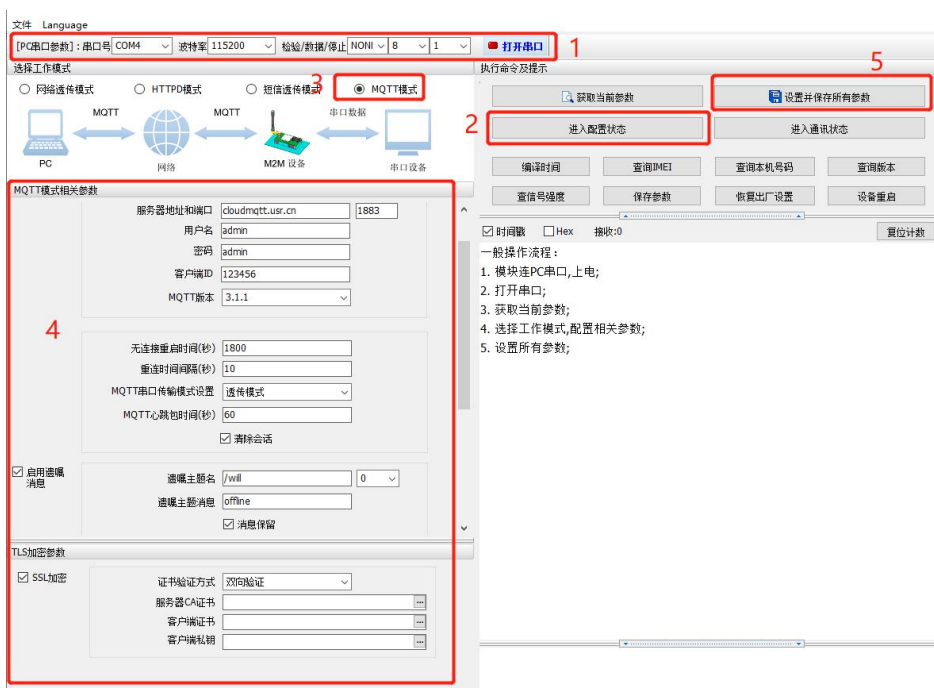
图 17. MQTT 模式通用接入方式示意图
