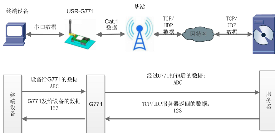
图 6. 网络透传模式
