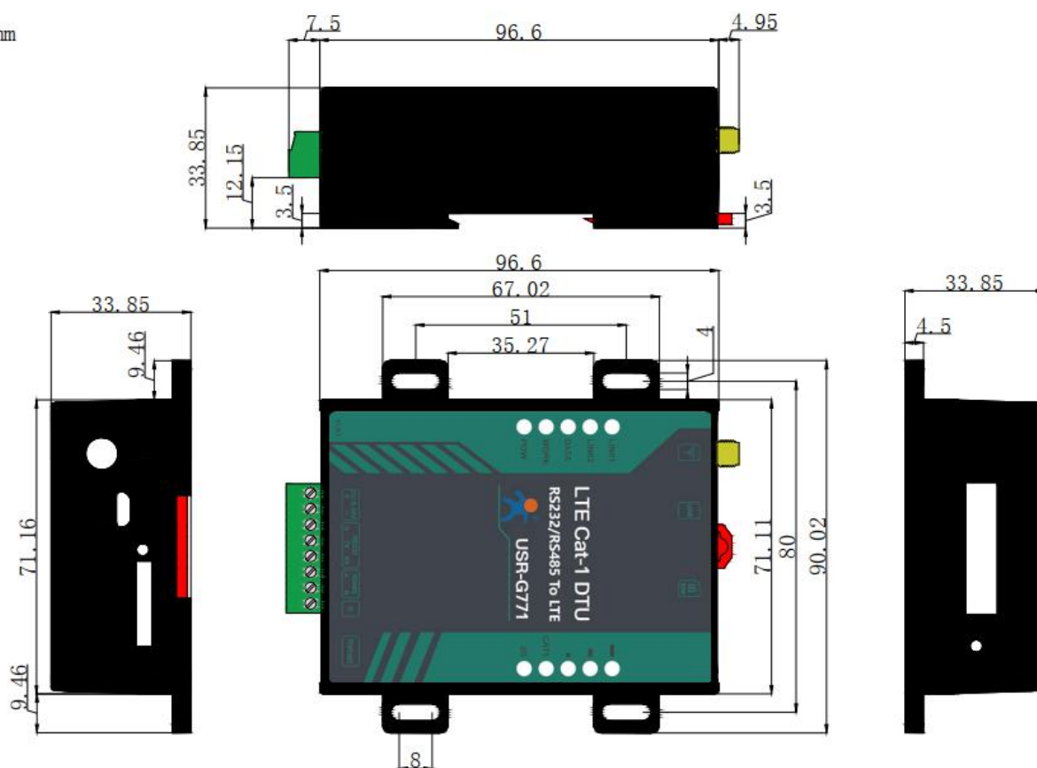
图 2. USR-G771 尺寸图
