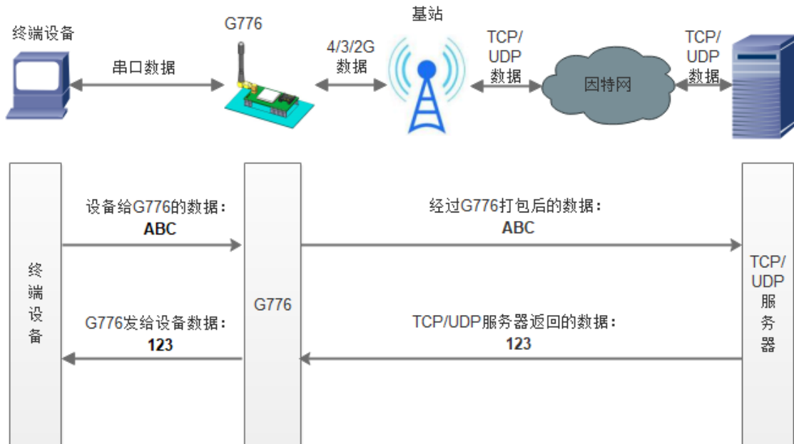
图 8 网络透传模式
