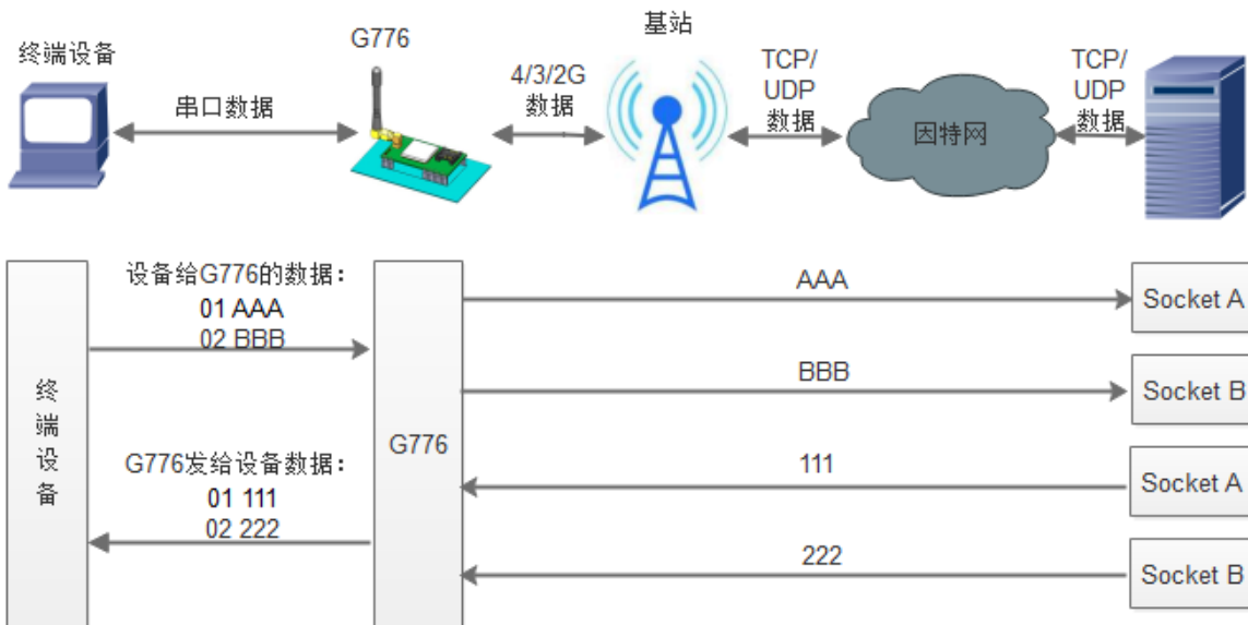
图 21 套接字分发协议示意图
