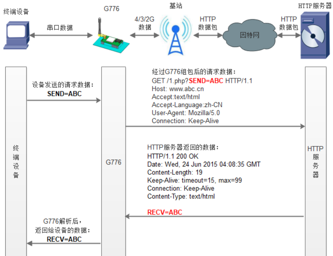
图 11 HTTPD 模式
