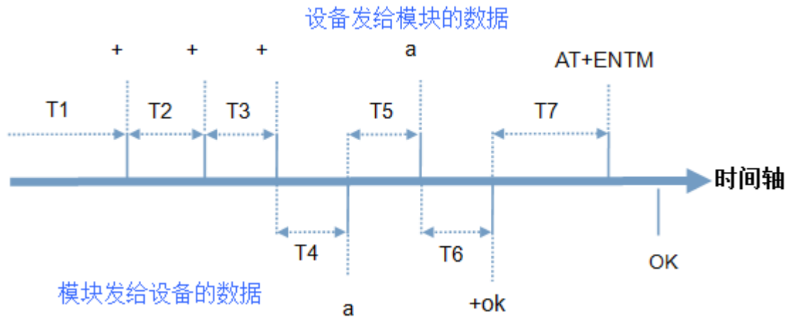
图 34 切换指令模式时序
