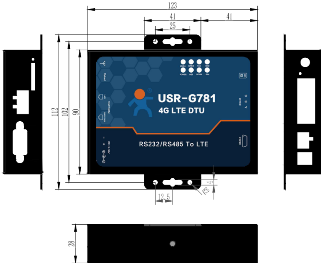
图 5 尺寸示意图
