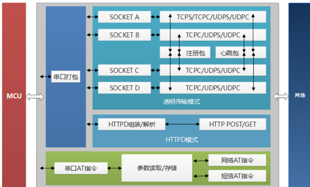
图 16 DTU 功能框图
