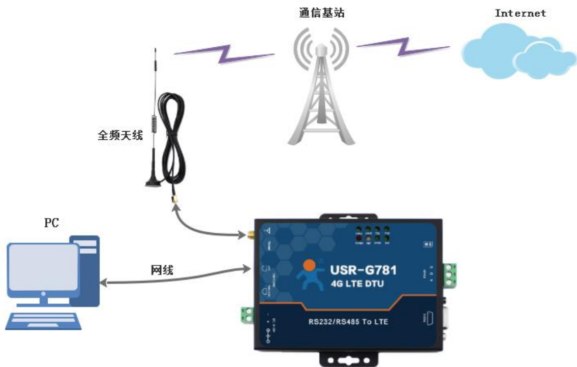
图 8 联网示意图
