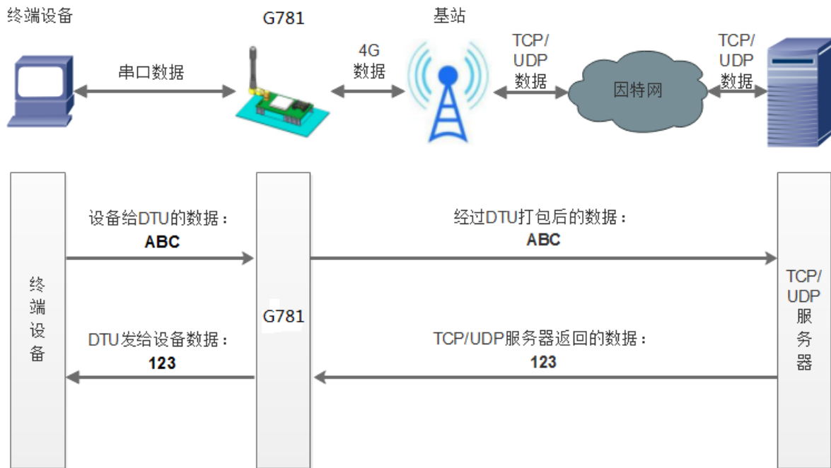
图 17 网络透传模式
