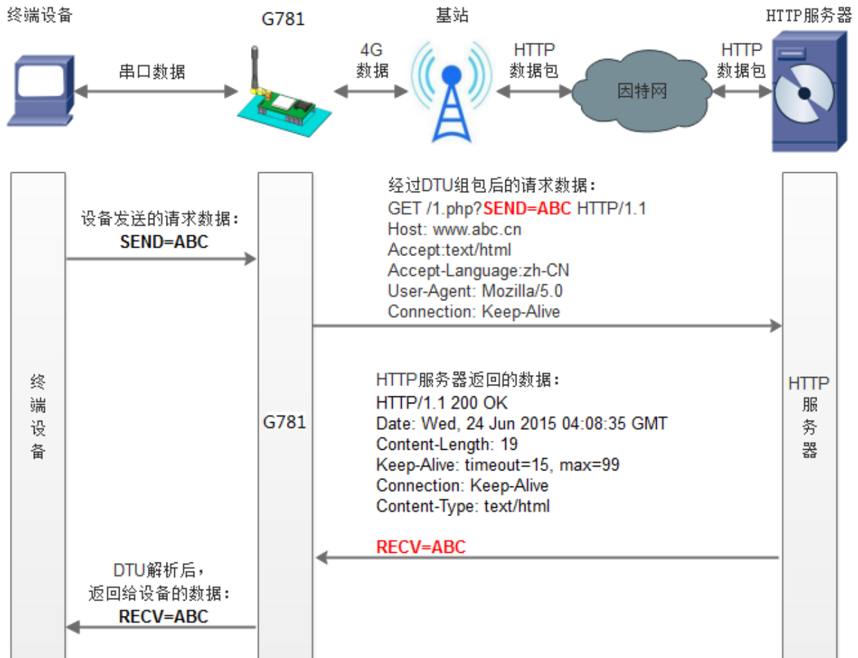
图 19 HTTPD 模式
