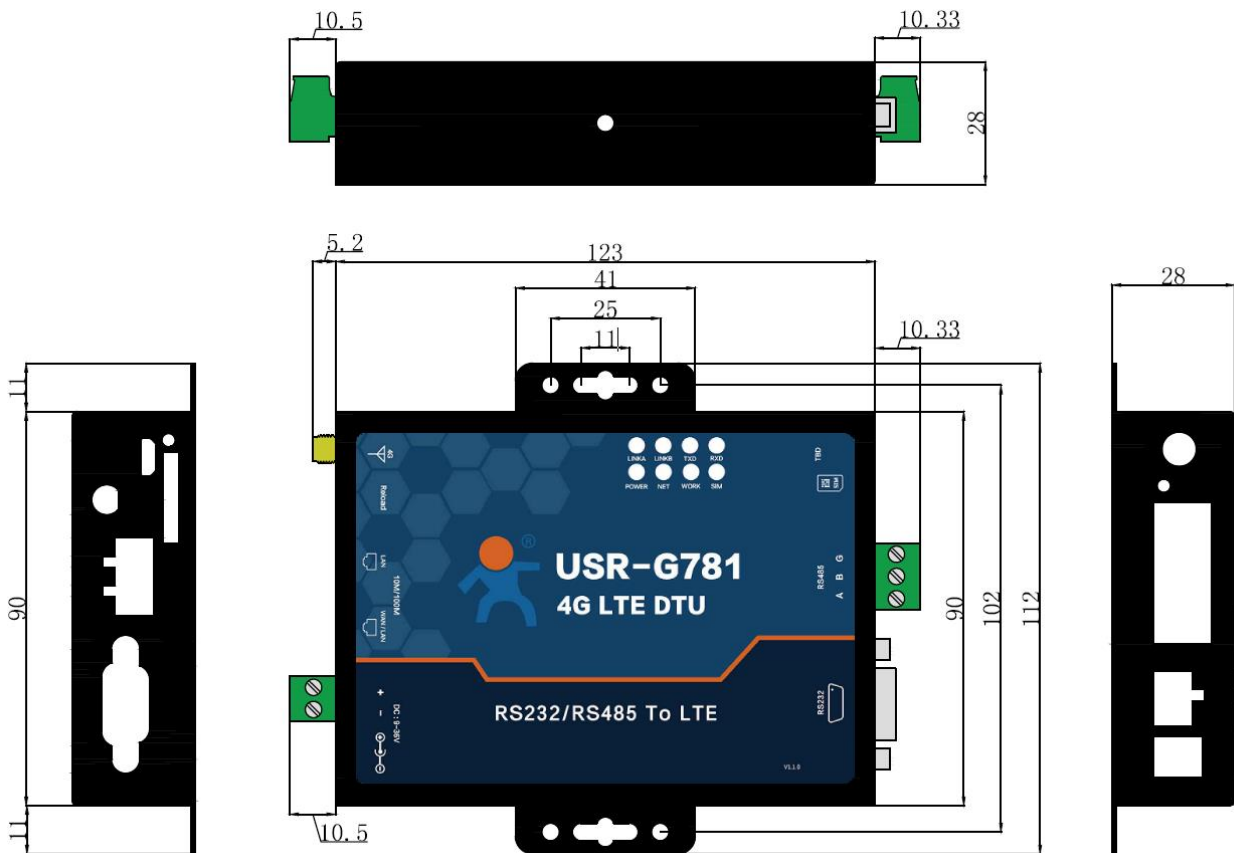
图 2 尺寸示意图
