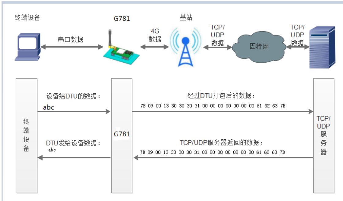
图 109 UDC 协议示意图
