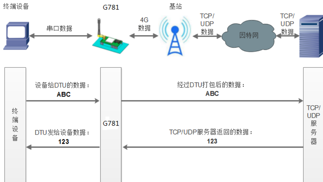
图 103 网络透传模式
