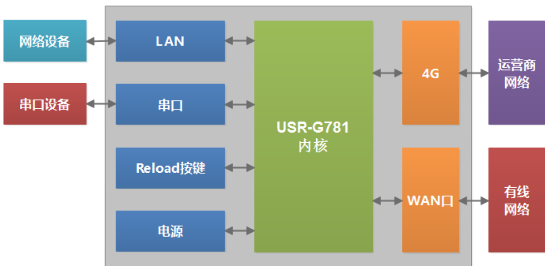
图 4 路由器功能框图
