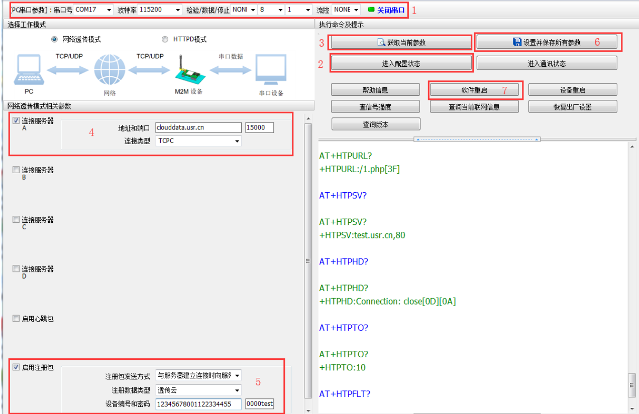
图 119 设置软件示意图
