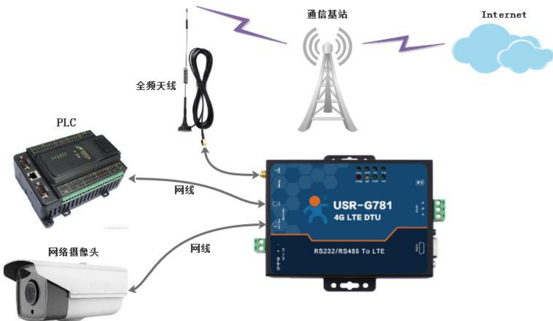
图 100 联网示意图
