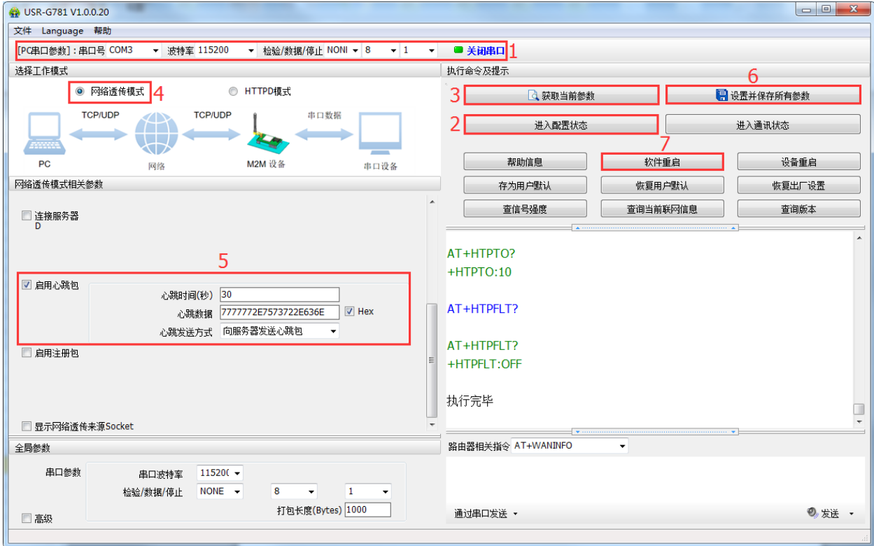
图 117 设置软件示意图
