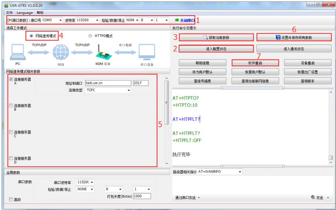
图 104 设置软件示意图
