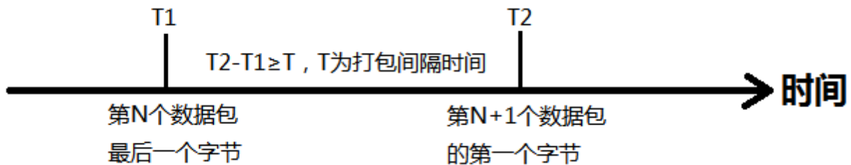
图 111 时间触发模式
