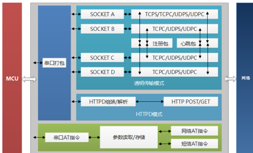
图 102 DTU 功能框图
