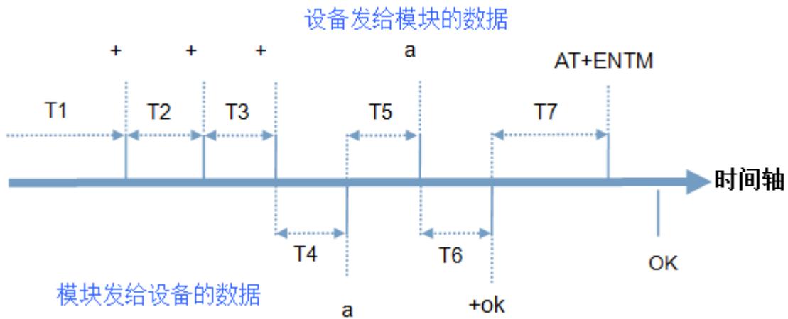
图 121 切换指令模式时序
