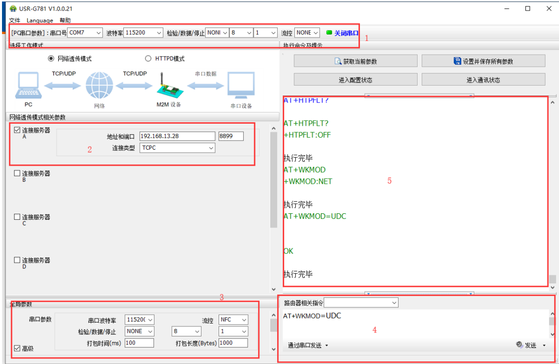
图 110 UDC 模式设置软件示意图
