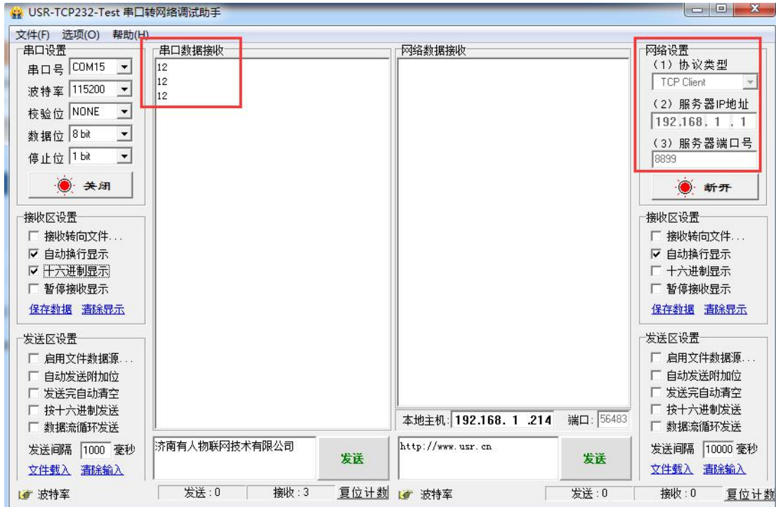
图 113 串口接收数据
