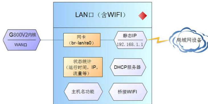
图 25 LAN 口功能示意图
