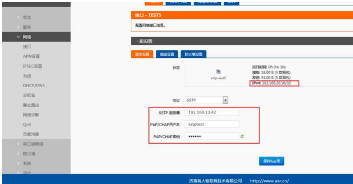
图 79 SSTP 基本设置
