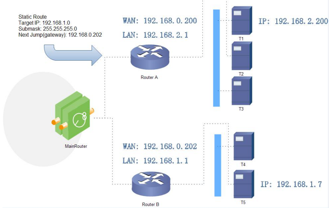
图 83 静态路由表实例图
