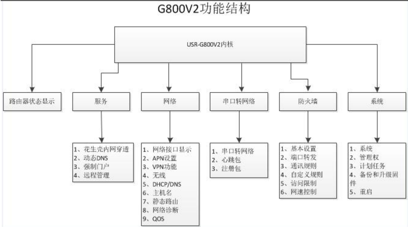
图 3 功能框图
