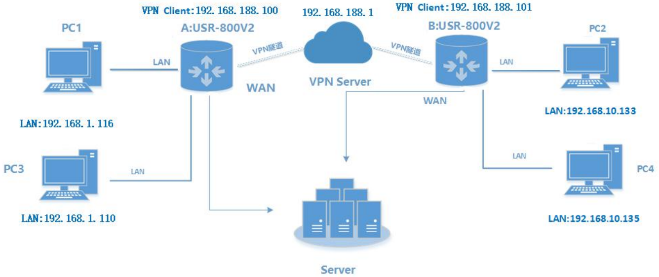
图 145 WAN+VPN+LAN 组网方式
