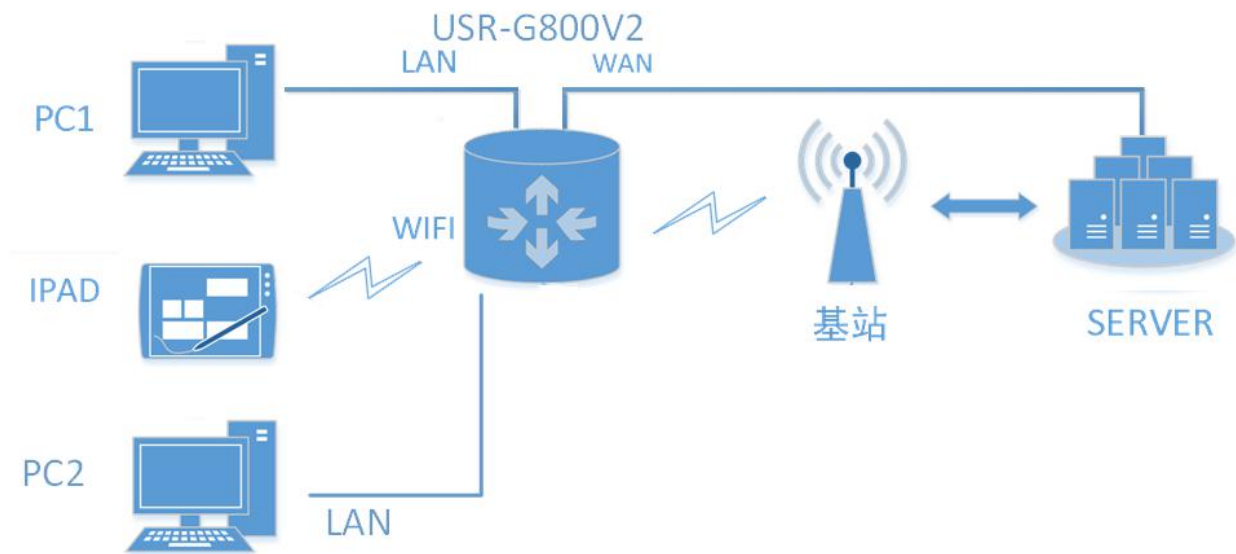
图 144 WAN 口加 4G 组网示意图
