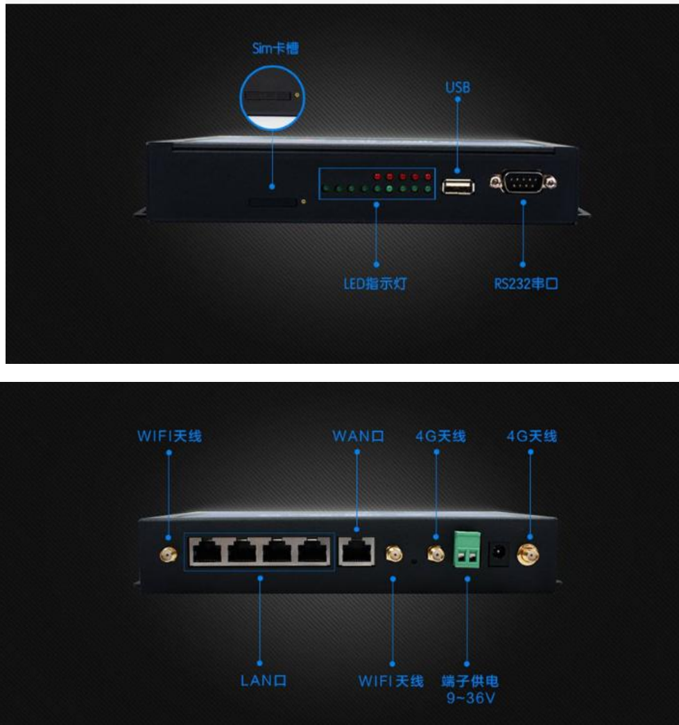
图 1 G800V2 接口图
