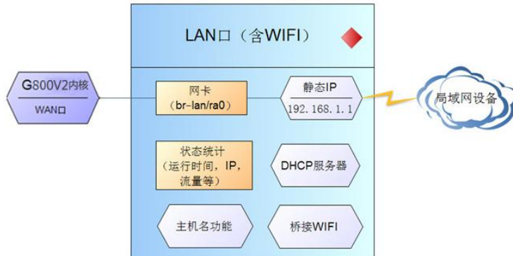
图 30 WIFI 功能示意图
