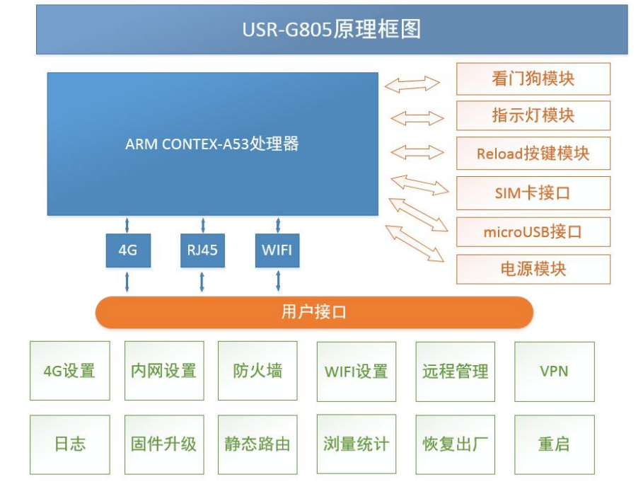
图 3 功能框图
