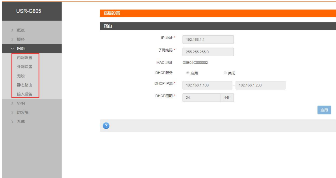
图 10 网络界面
