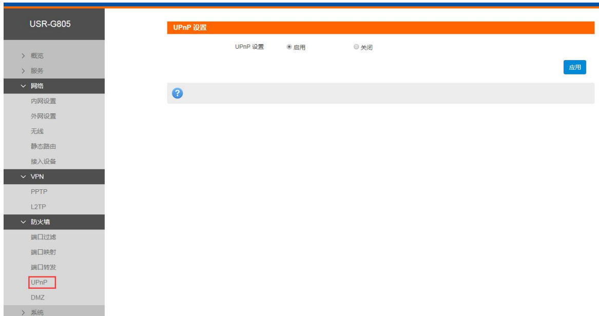
图 63 UPnP 页面
